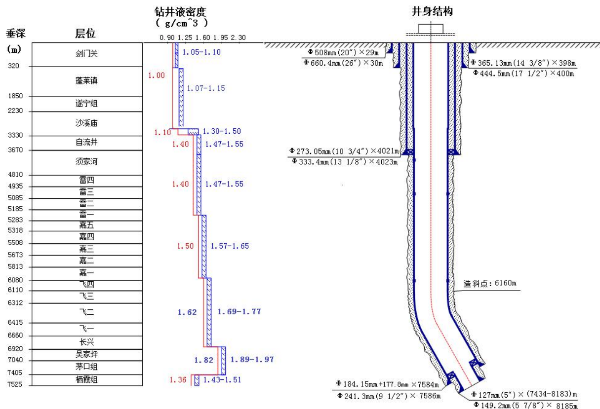
图 5.3-1 双鱼 001-X7 井钻井井身结构示意图
