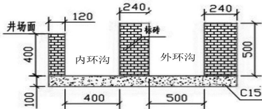
图 5.2-2 井场雨污分流排水沟结构图
