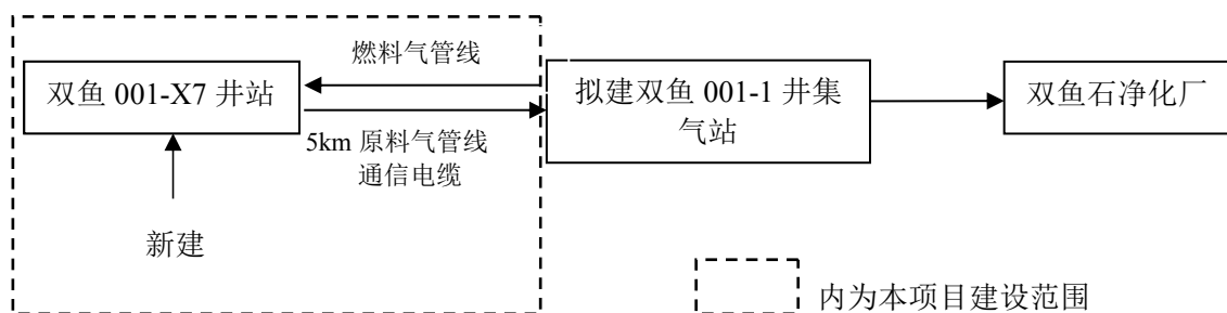
图 5-9 本项目集输示意图
