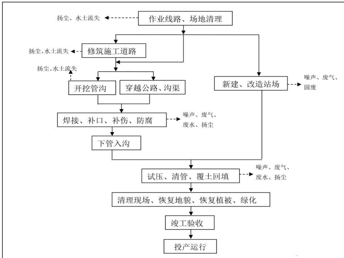
图 5-1 地面集输工程施工期施工工艺流程图
