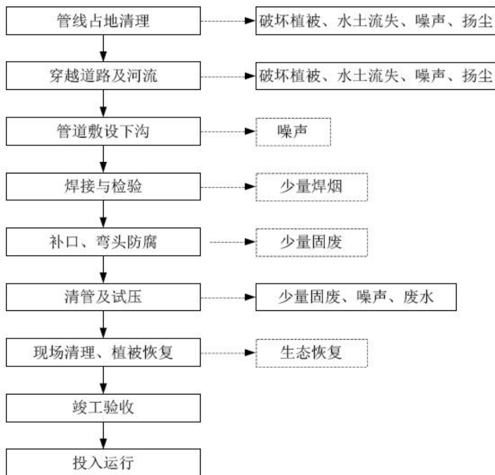
图 5-2 项目管道施工流程及产污位置图
