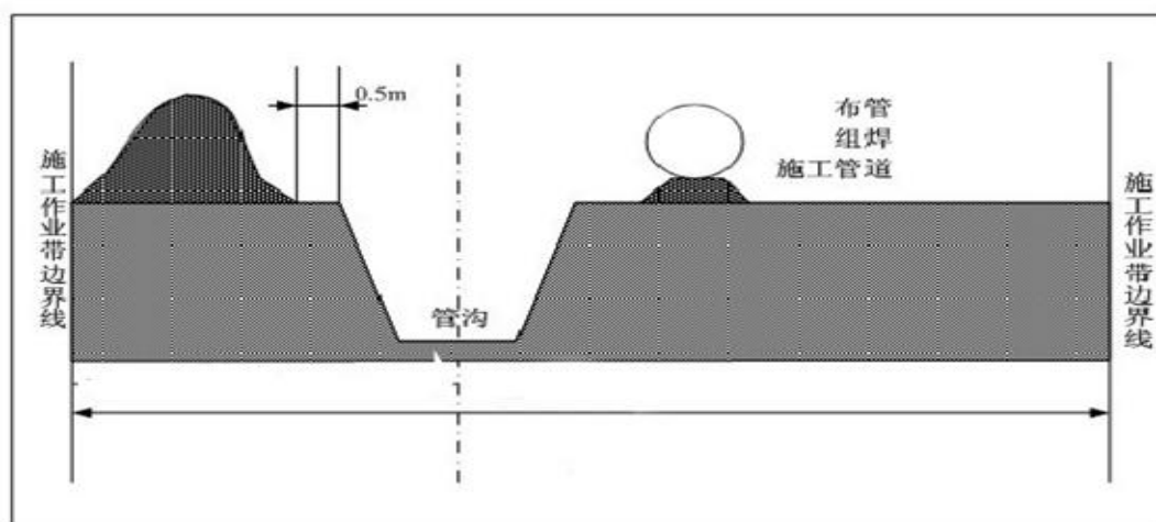
图 5-3 管段施工方式断面示意图
