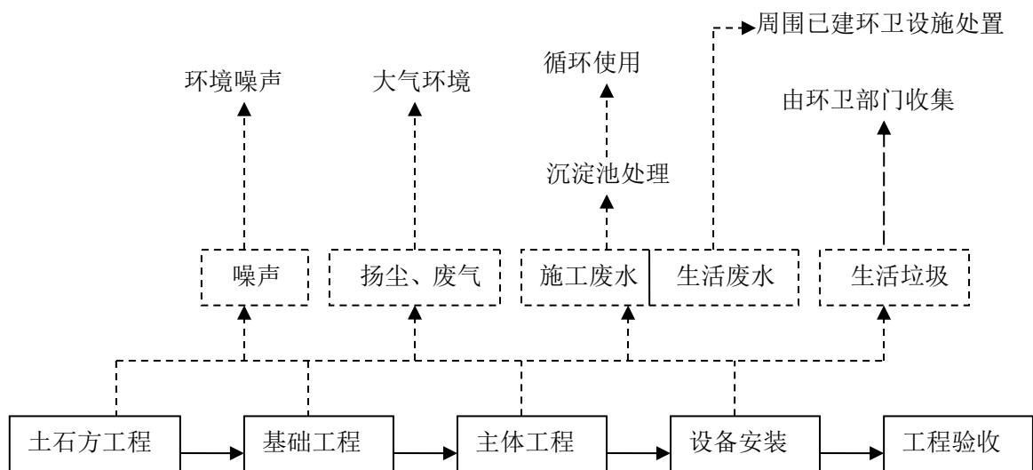
图 5-8 新建站场施工流程及产污位置图
