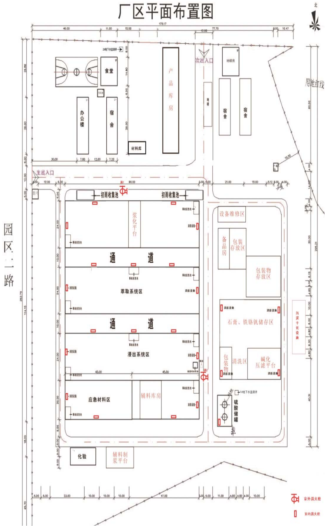
图 3.2-1 场地平面布置图
