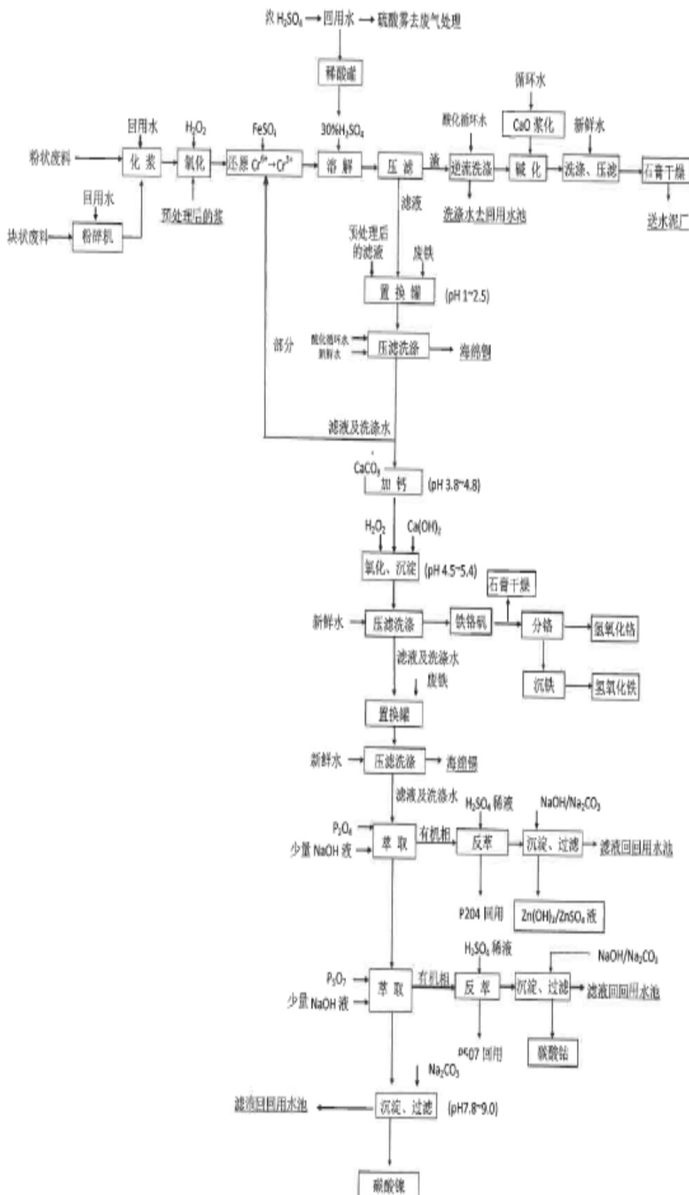
图 3.2-3 金属回收生产线工艺流程及产物环节
