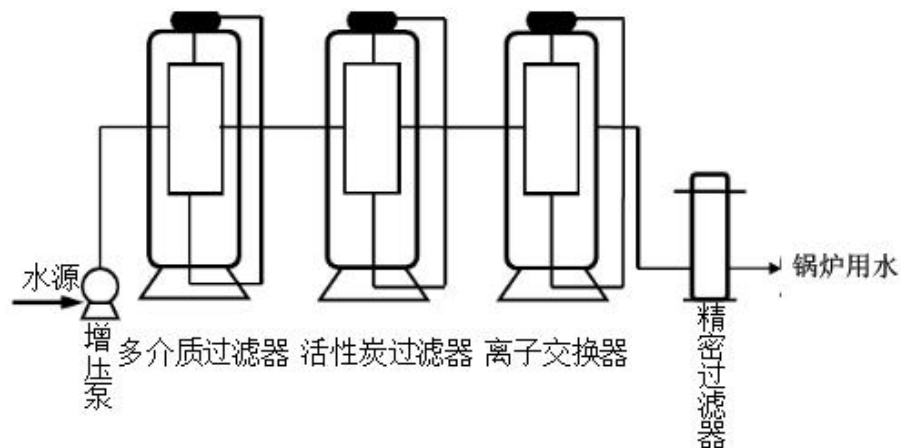
图 1-3 软水生产工艺流程图
