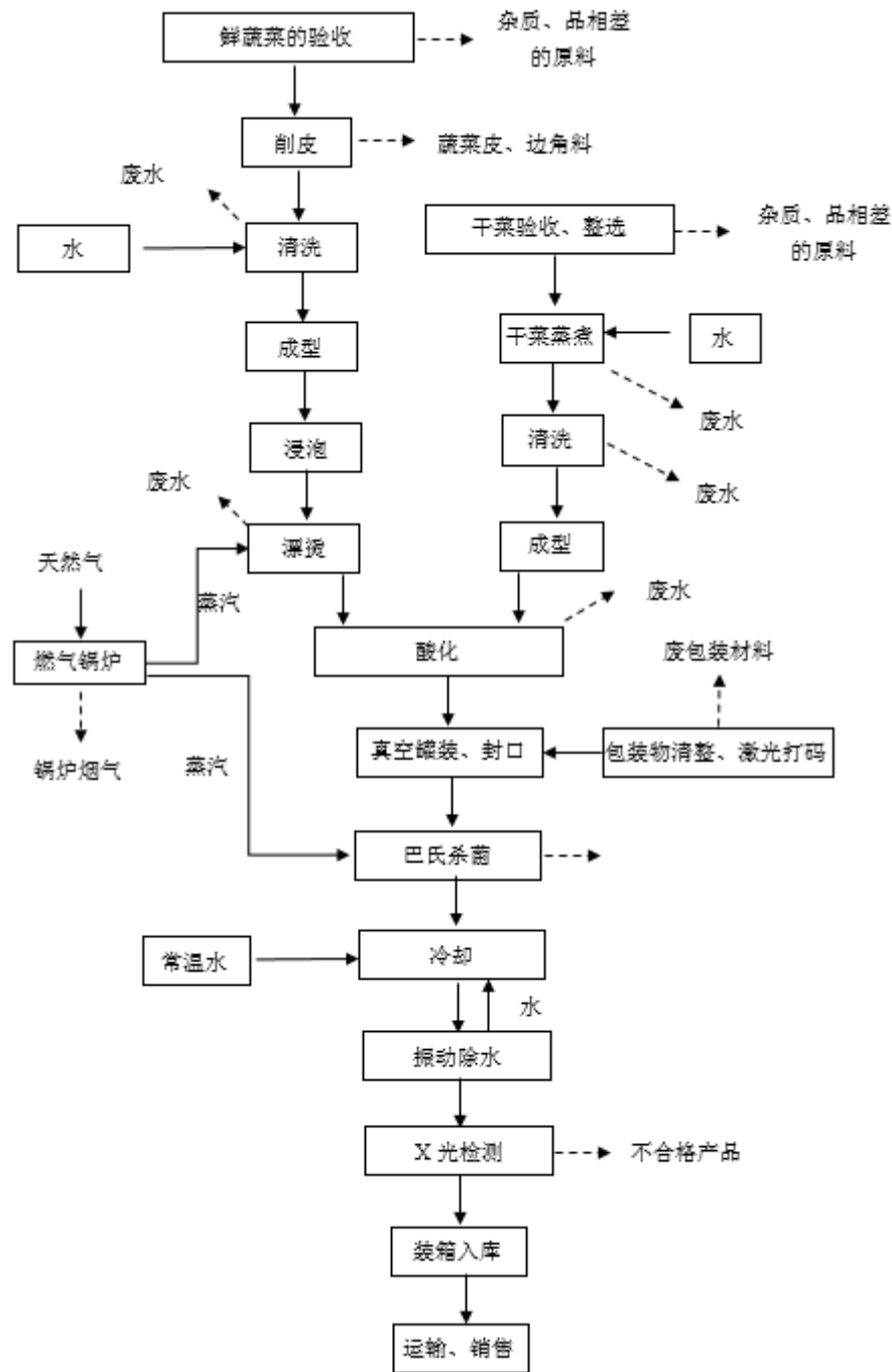
图 1-3 其蔬菜包系列生产工艺流程及产污环节图
