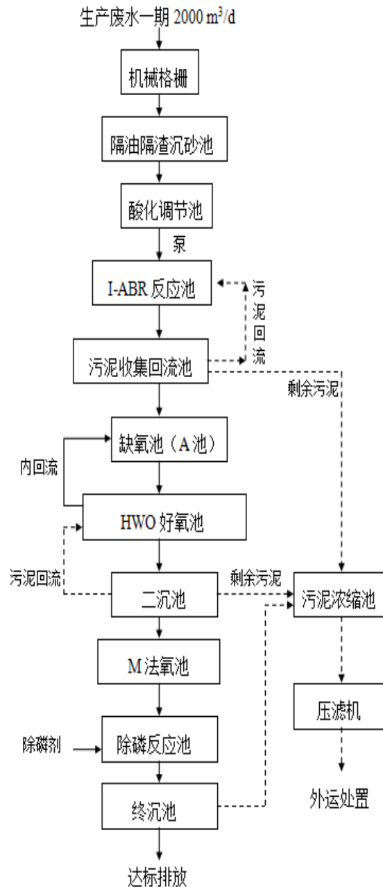
图 1-4 本项目污水处理流程图
