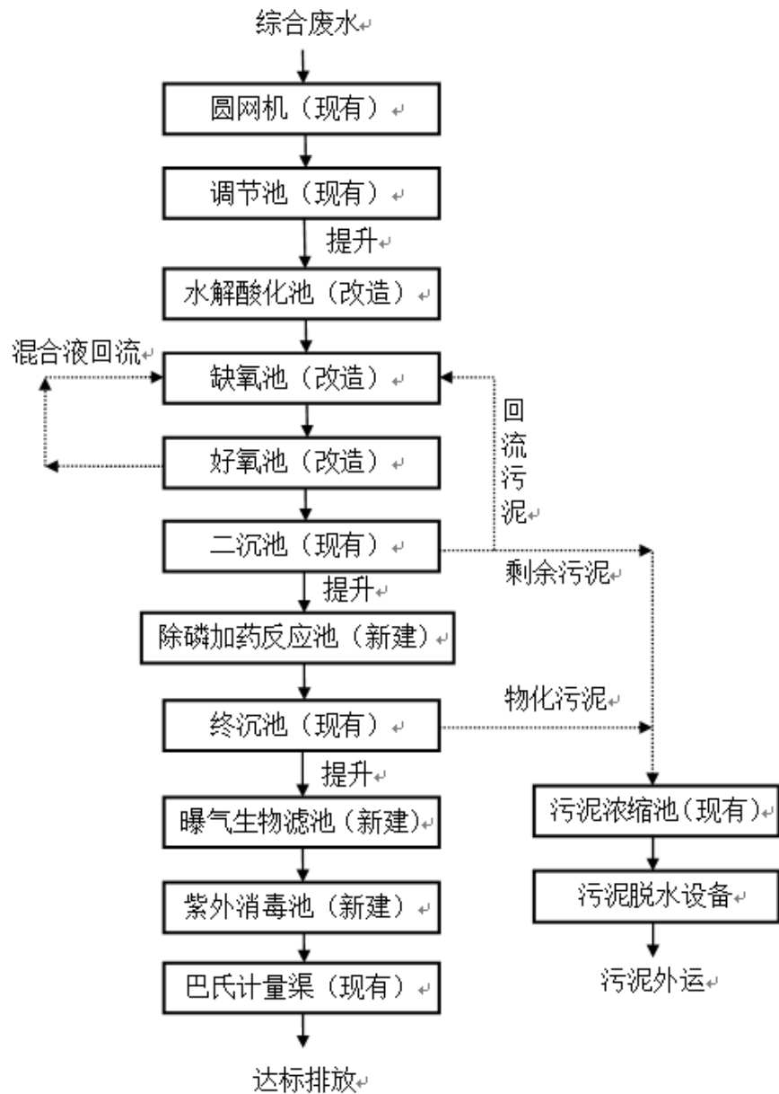
图 5-10 园区污水处理厂污水处理流程图
