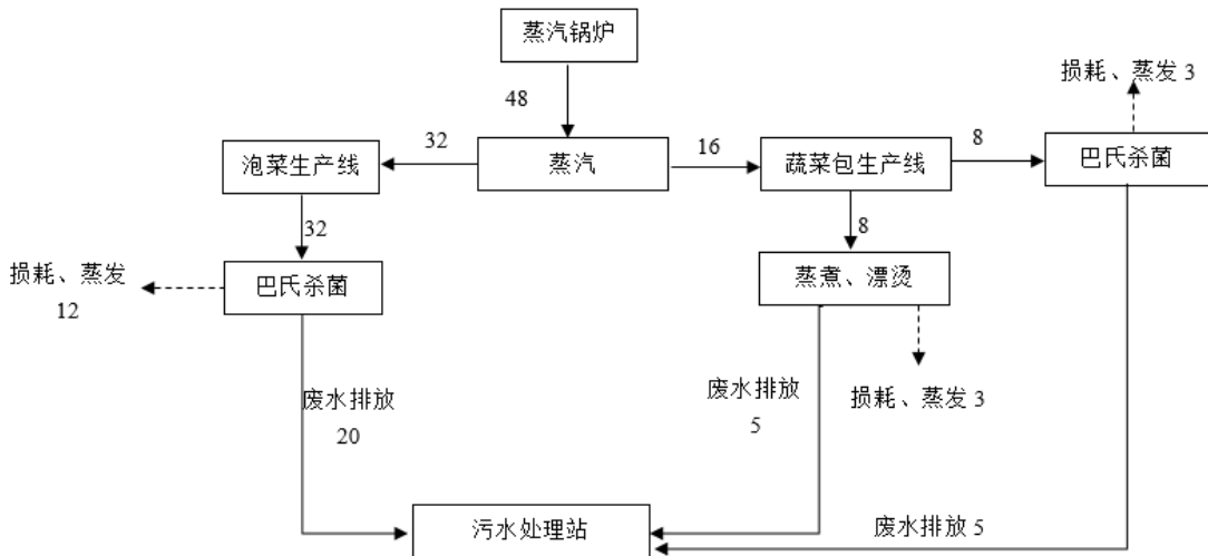
图 5-7 本项目蒸汽平衡图 t/d
