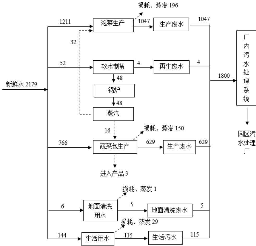
图 5-6 本项目水平衡图 m^3/d
