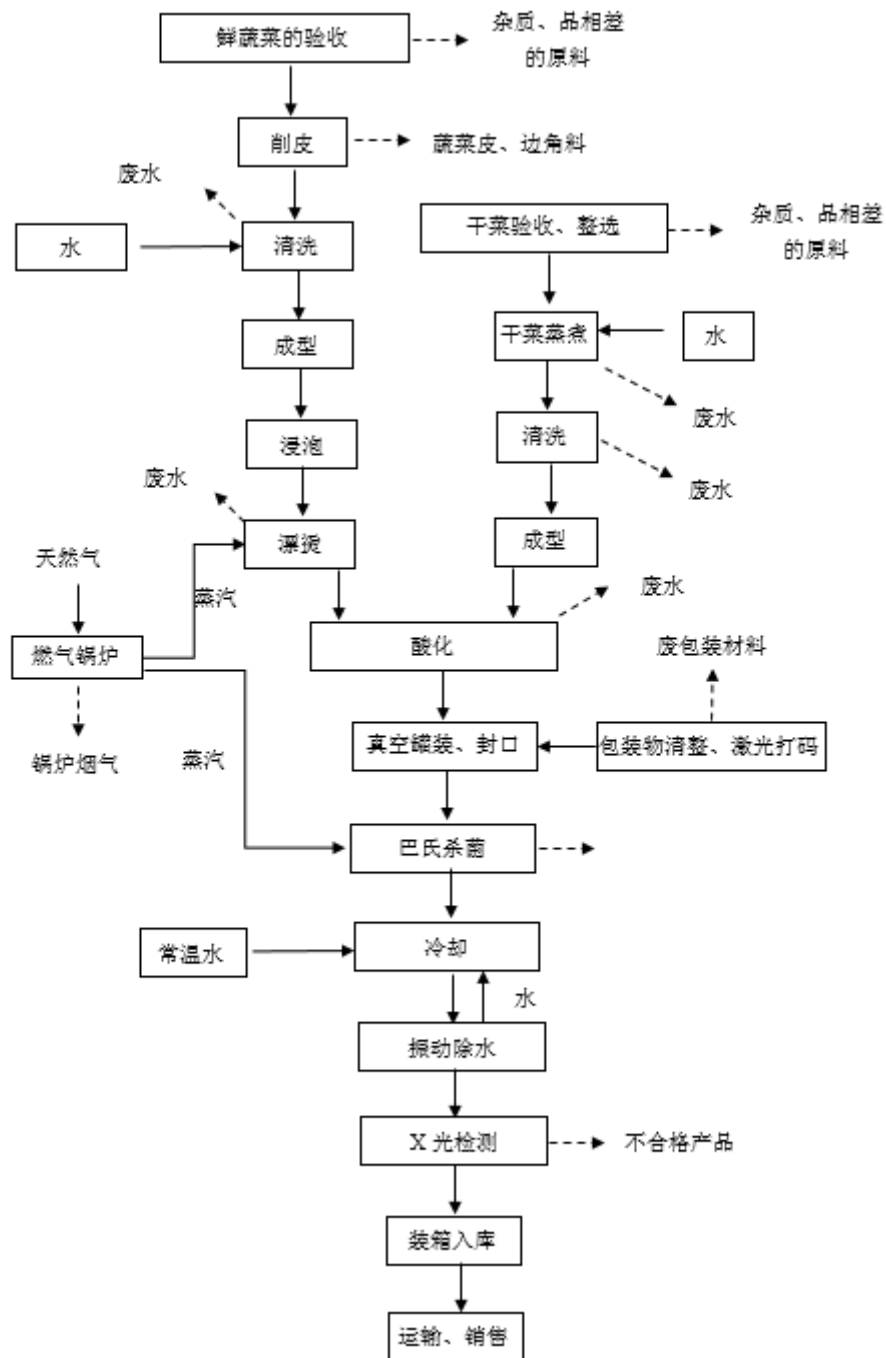
图 5-3 其他食品（蔬菜包系列）生产工艺流程及产污环节图
