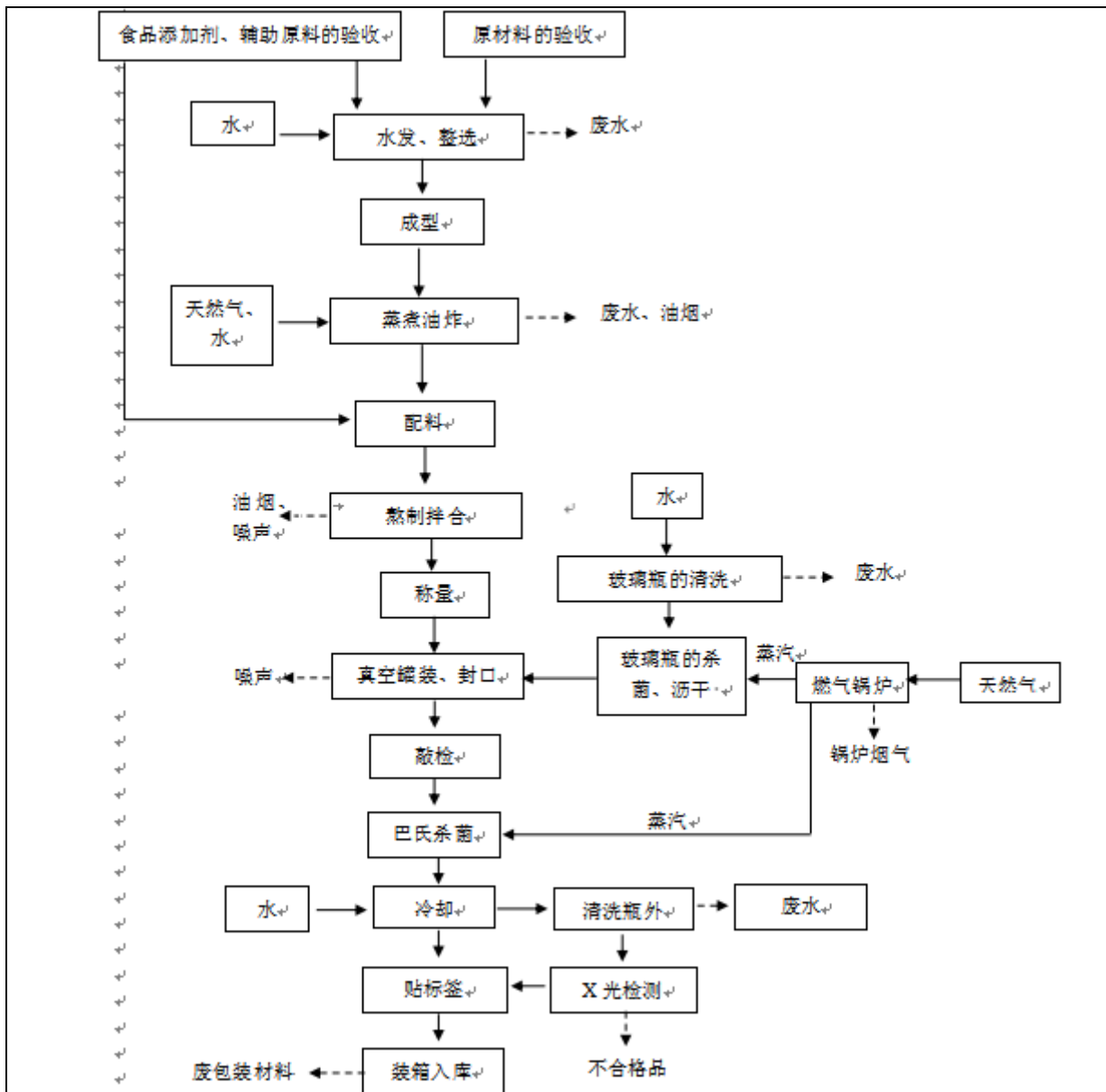
图 5-2 瓶装调味品生产工艺流程及产污环节图
