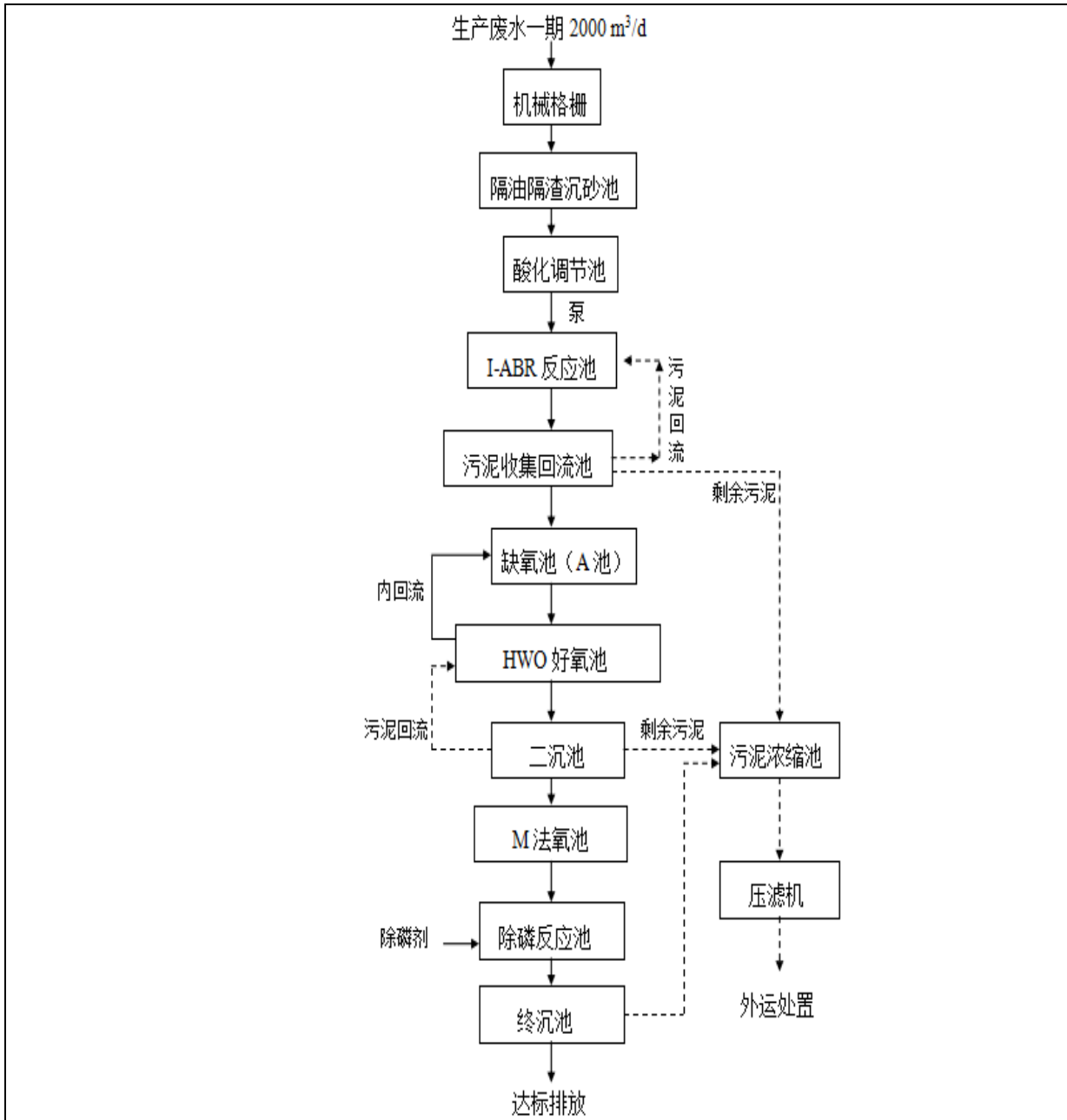
图 5-9 本项目污水处理流程图
