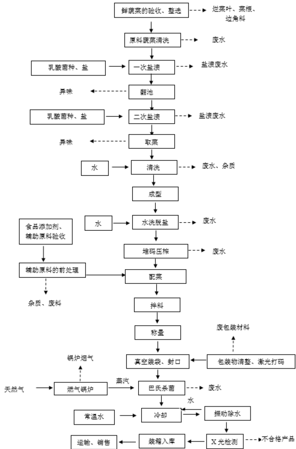
图 1-2 袋装泡菜生产工艺流程及产污环节图
