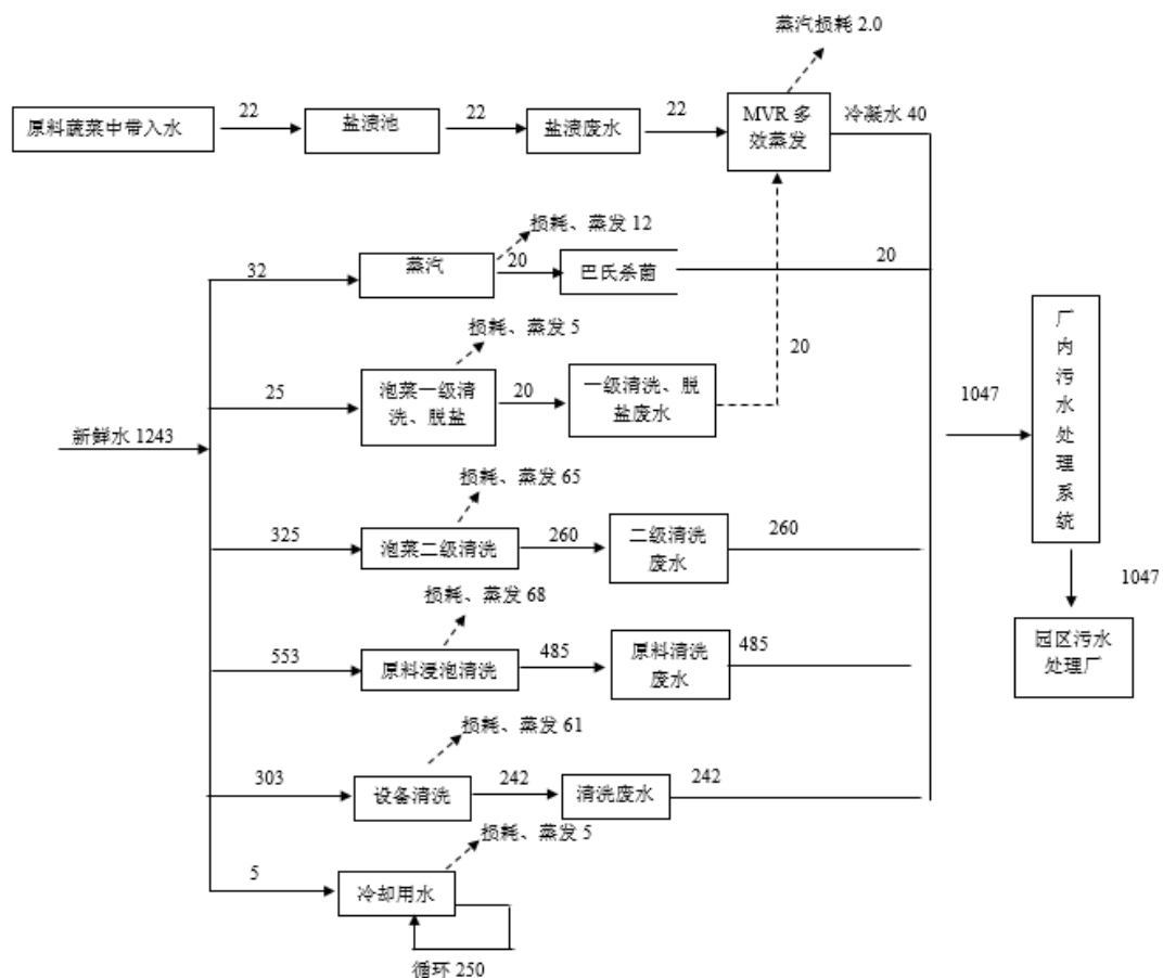
图 5-4 调味品生产线水平衡图 m 3 /d
