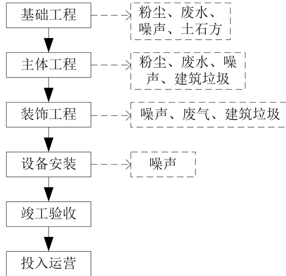
图 5-1 施工期工艺流程及产污位置图
