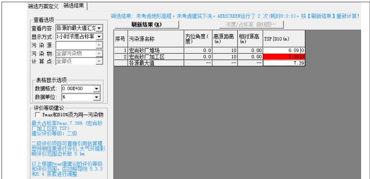
图 7-1 大气预测结果图
