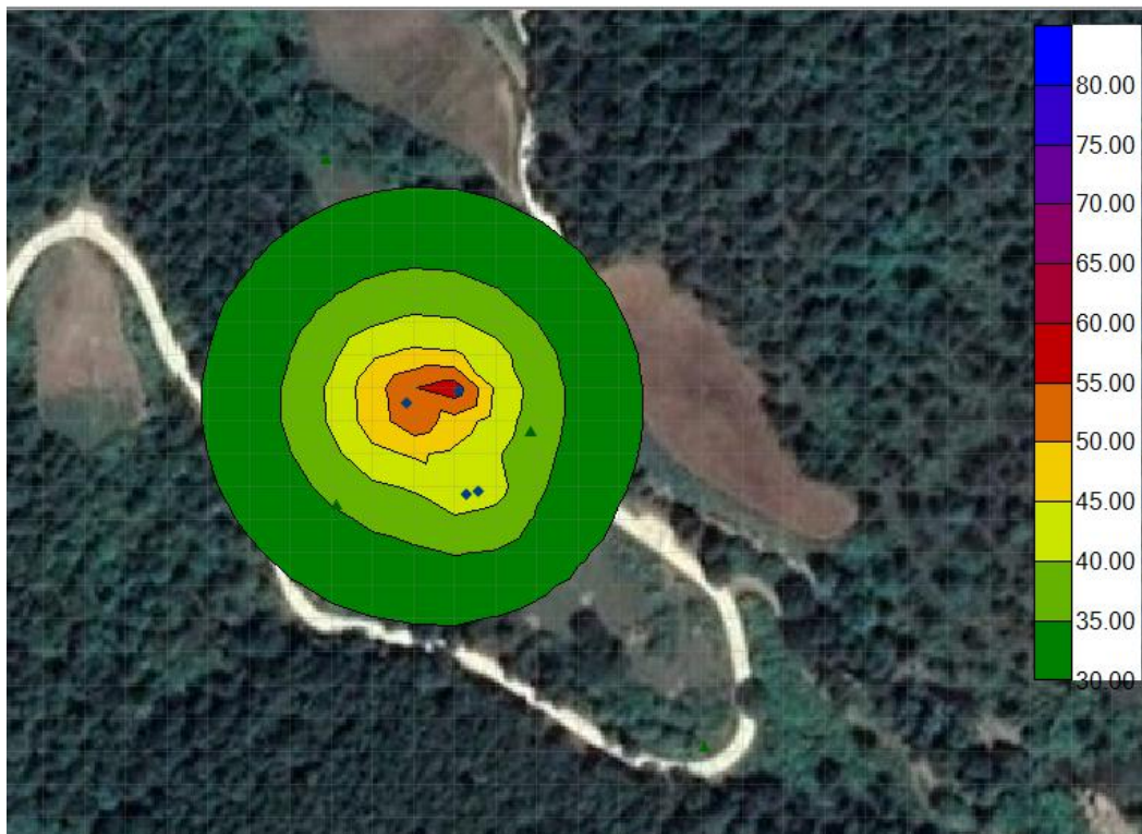
图 7-2 项目等声值线图
