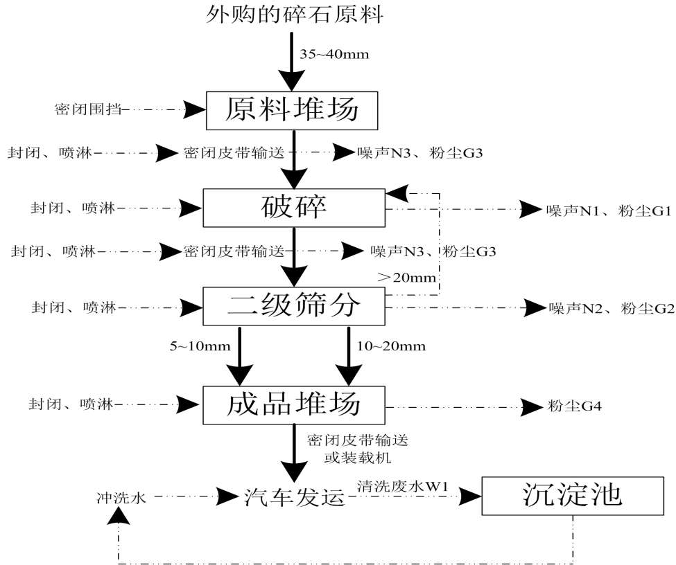
图 5-2 本项目运营期生产工艺流程图
