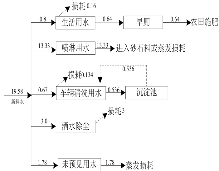
图 1-3 项目水平衡及废水处理图 单位：m 3 /d
