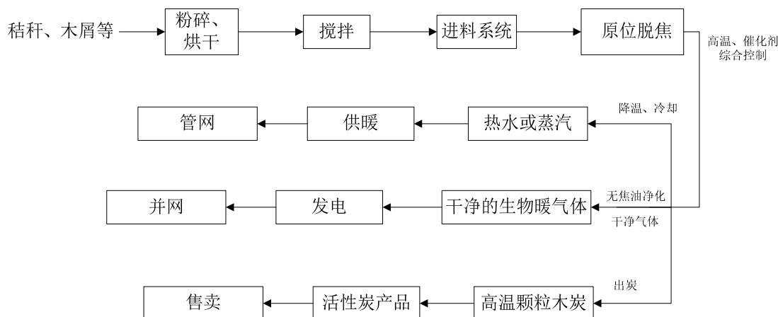
图 2.4-5 项目工艺流程图
