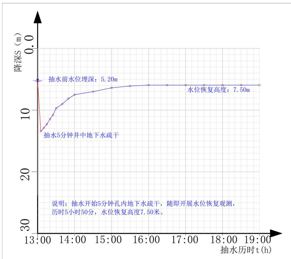
图 3.1-7 现场含水层抽水试验 S-t 关系曲线图
