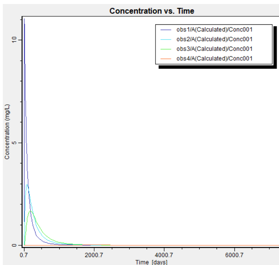
图 5.7-5 非正常状况主径流方向下游 COD Mn 浓度随时间变化曲线 (20m、40m、60m、居民点)
