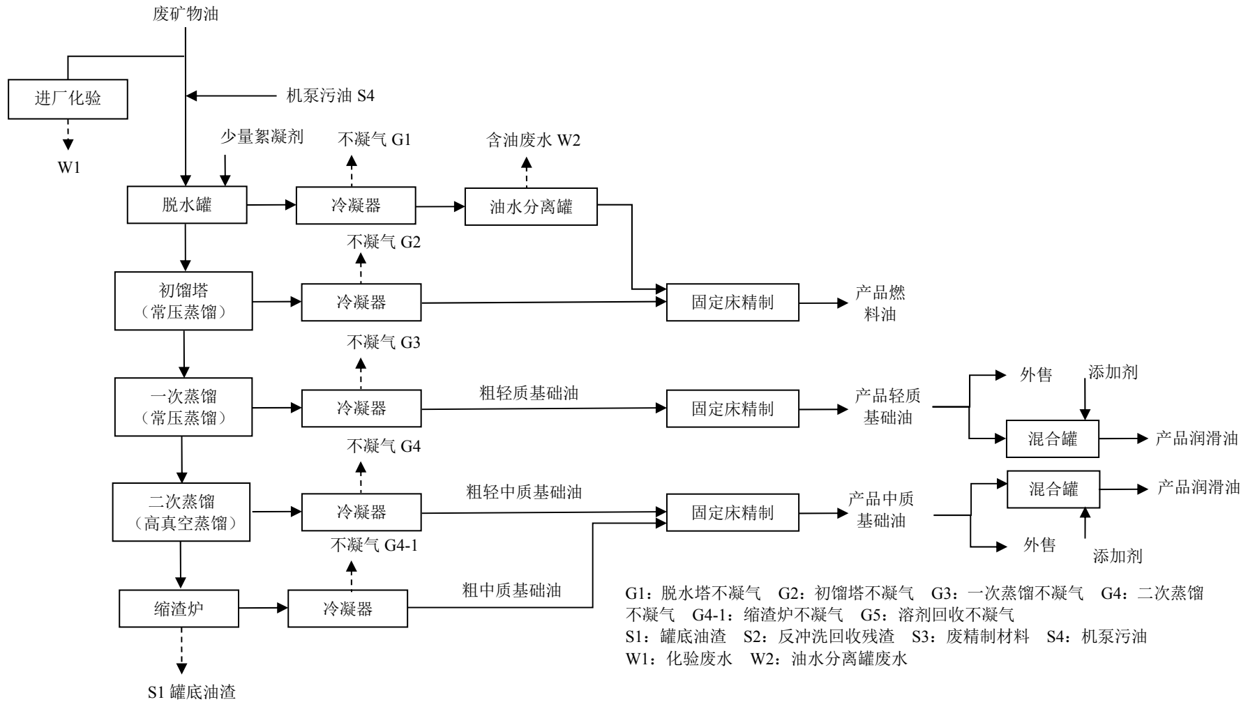
图 2.4-10 节能环保产业典型生产工艺流程图（废油回收）
