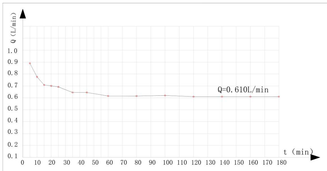
图 3.1-6 现场包气带渗水实验 Q-t 关系曲线图
