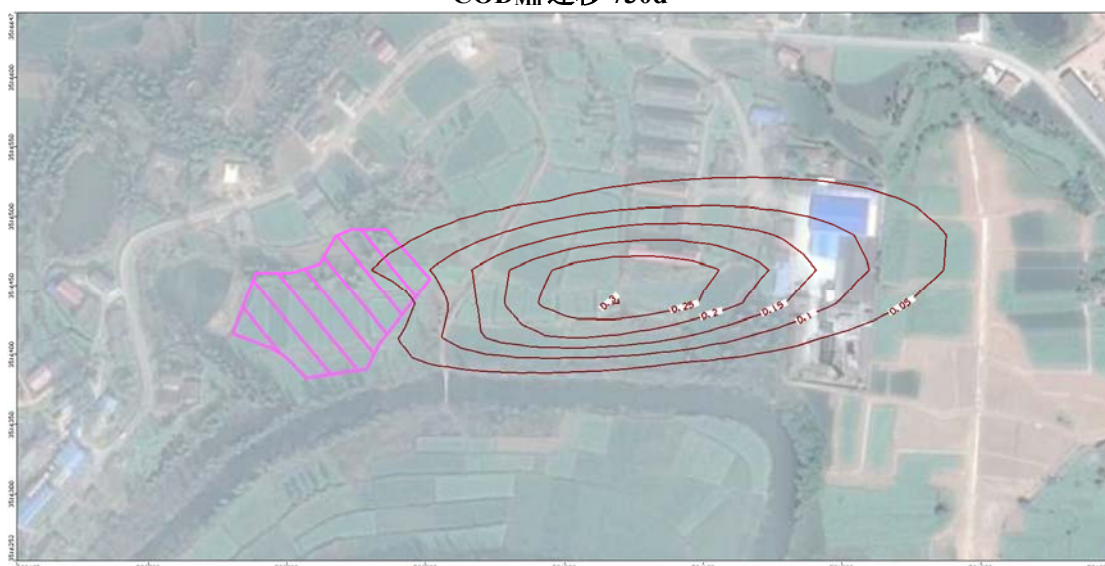
COD Mn 迁移 1000d
