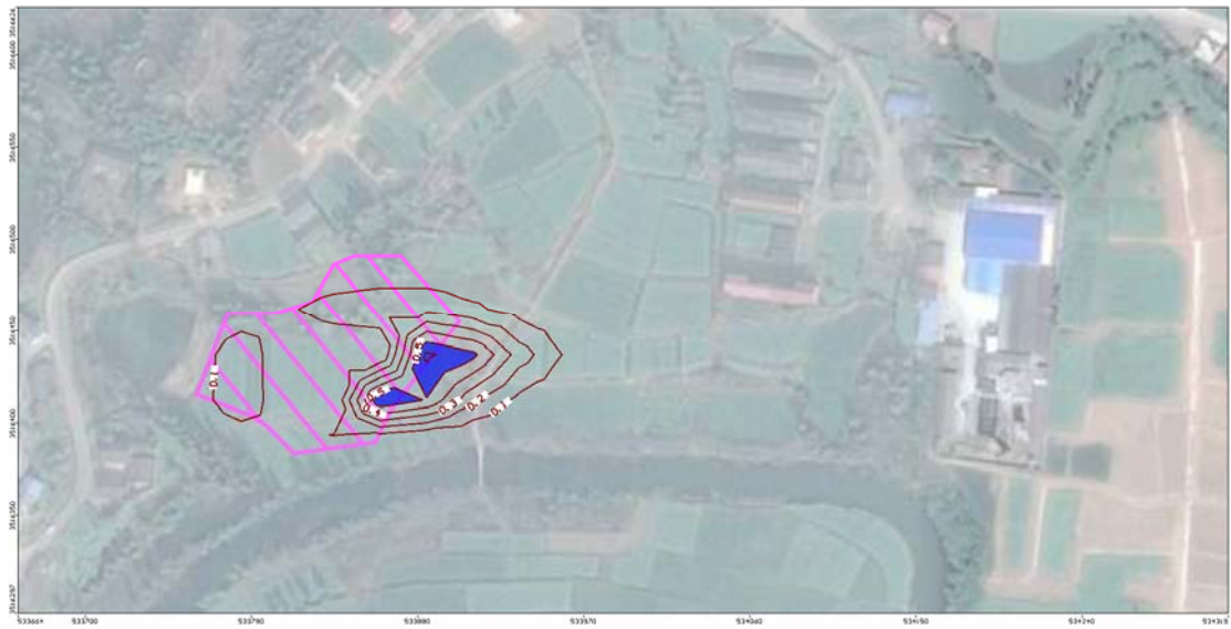
NH 3 -N 迁移 100d
