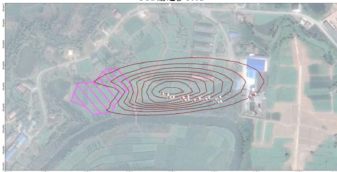
COD Mn 迁移 730d
