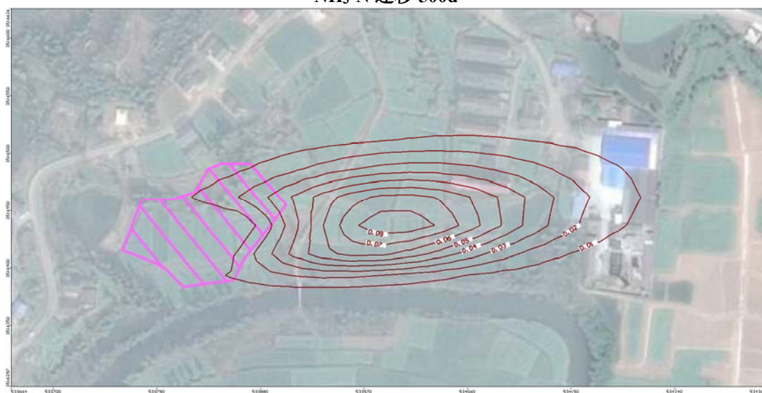
NH 3 -N 迁移 730d
