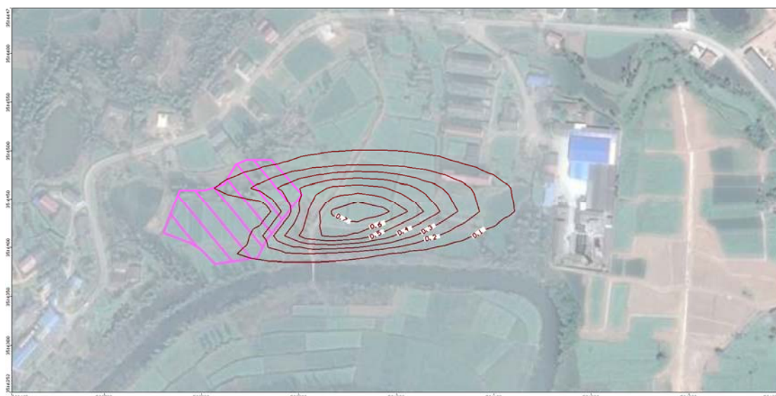
COD Mn 迁移 500d
