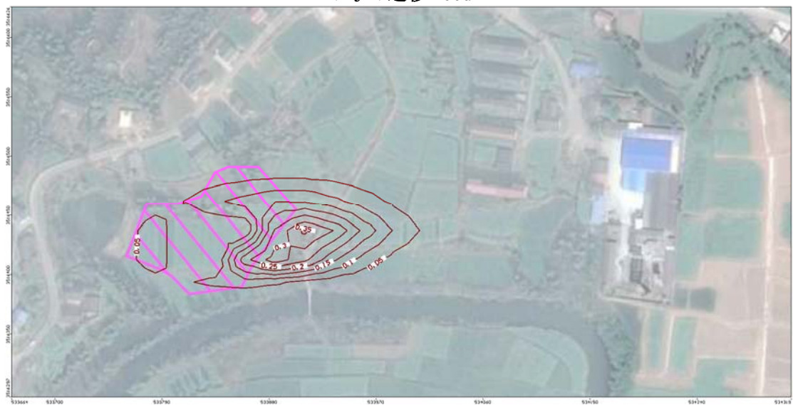
NH 3 -N 迁移 200d
