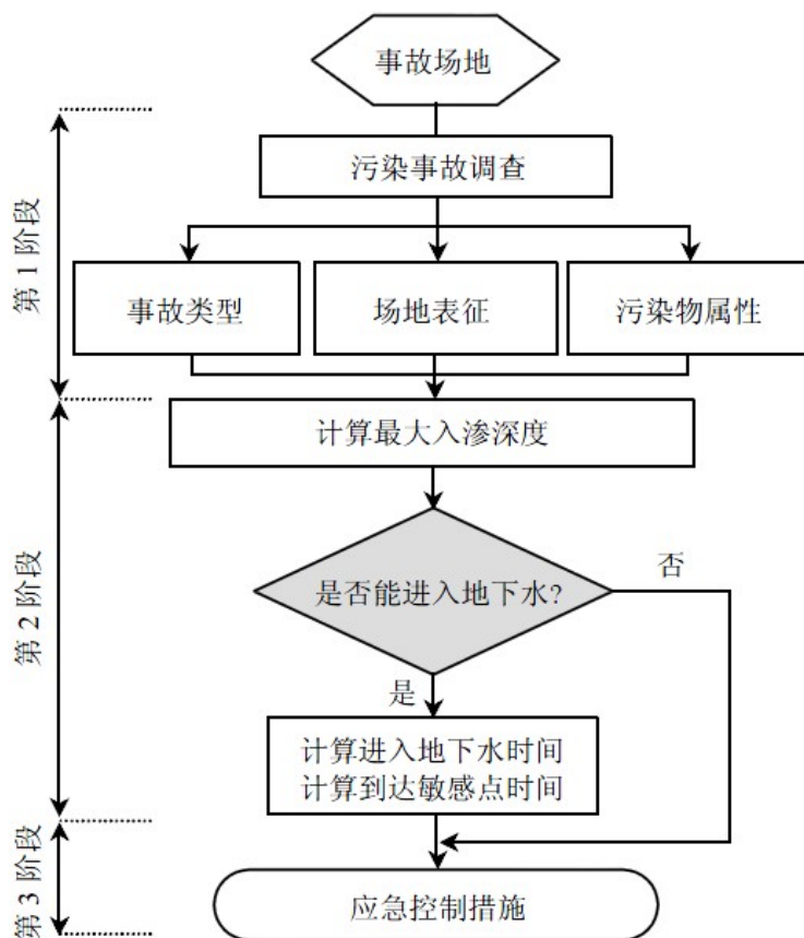
图 7.2-3 地下水污染风险快速评估与决策过程
