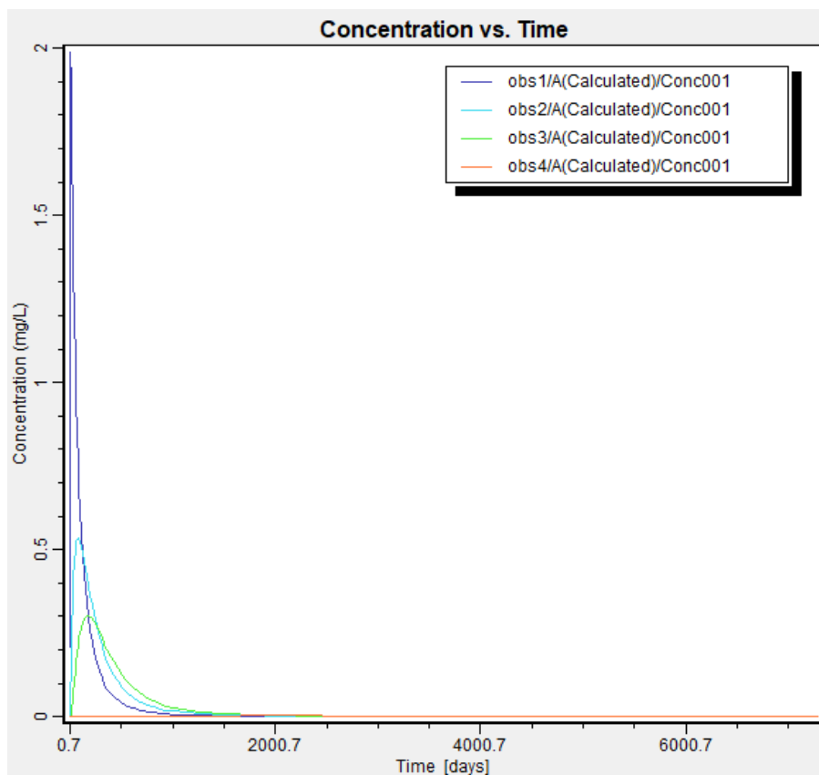
图 5.7-7 非正常状况主径流方向下游 NH 3 -N 浓度随时间变化曲线 (20m、40m、60m、居民点)
