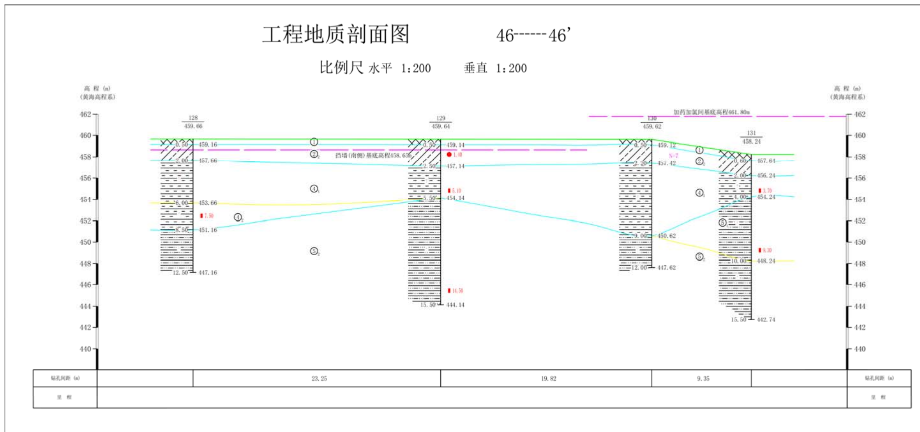
图 3.1-2 项目场地地质勘察 46-46'工程地质剖面图
