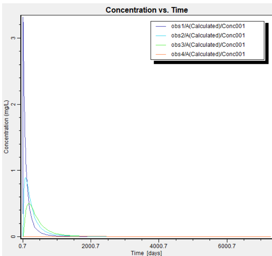
图 5.7-9 非正常状况主径流方向下游 TN 浓度随时间变化曲线 (20m、40m、60m、居民点)
