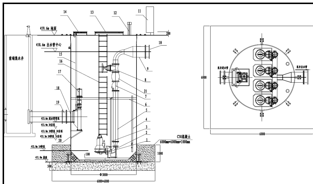
图 2.7-1 项目一体化泵站平面布置图
