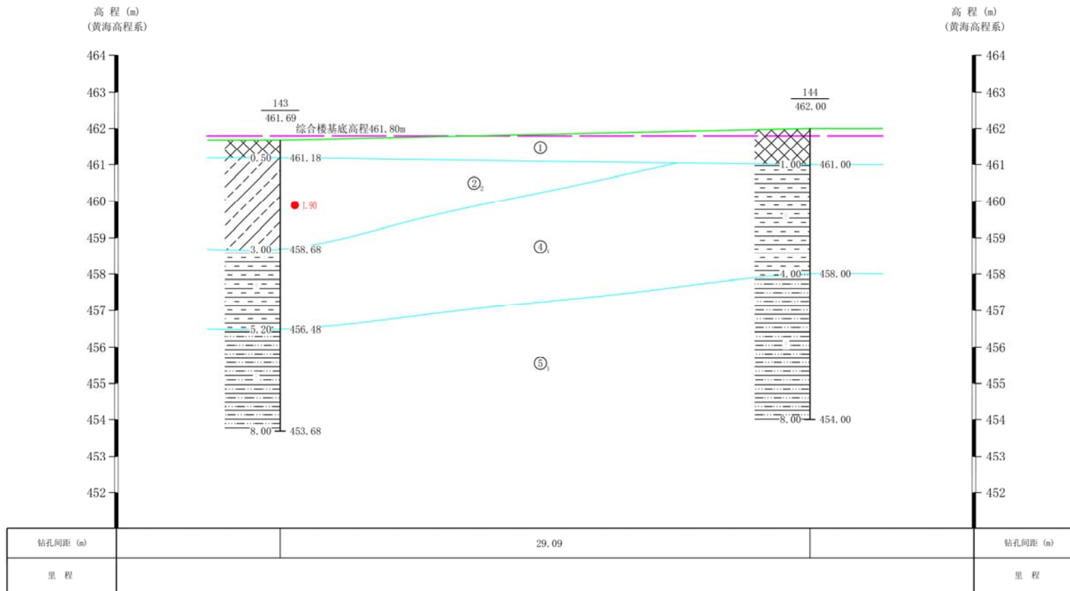
图 3.1-3 项目场地地质勘察 59-59'工程地质剖面图
