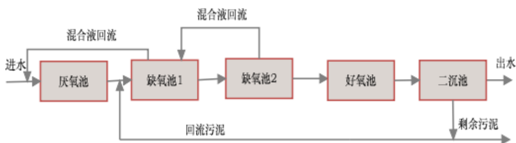
图 7.2-1 改良 A 2 /O 工艺流程框图
