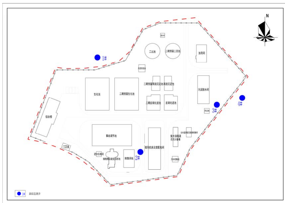
图 7.2-2 本项目跟踪监测井位置示意图
