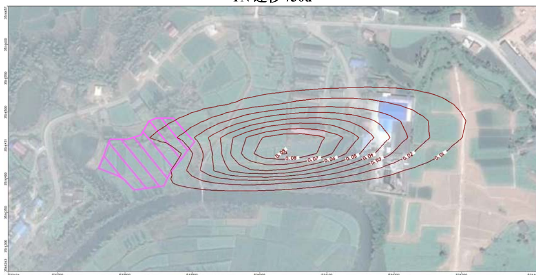
TN 迁移 1000d
