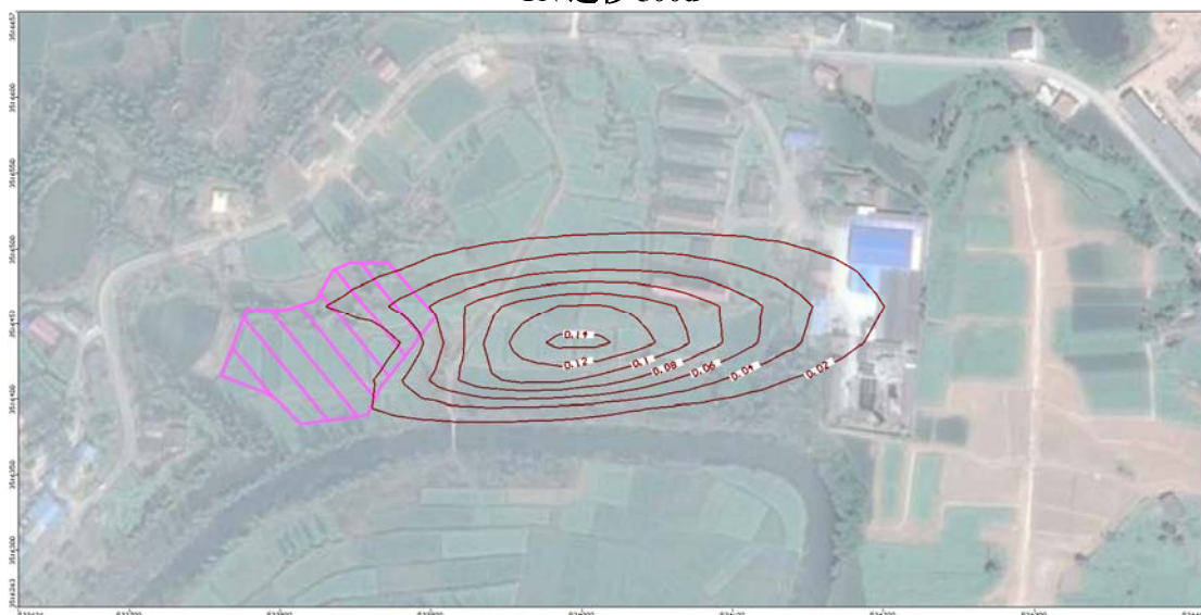
TN 迁移 730d
