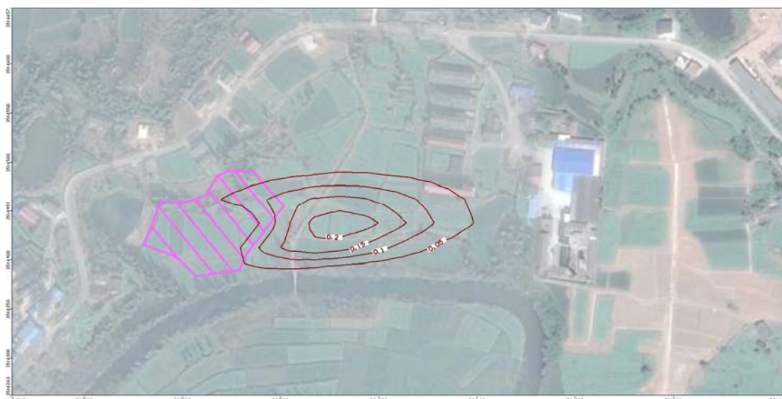
TN 迁移 500d
