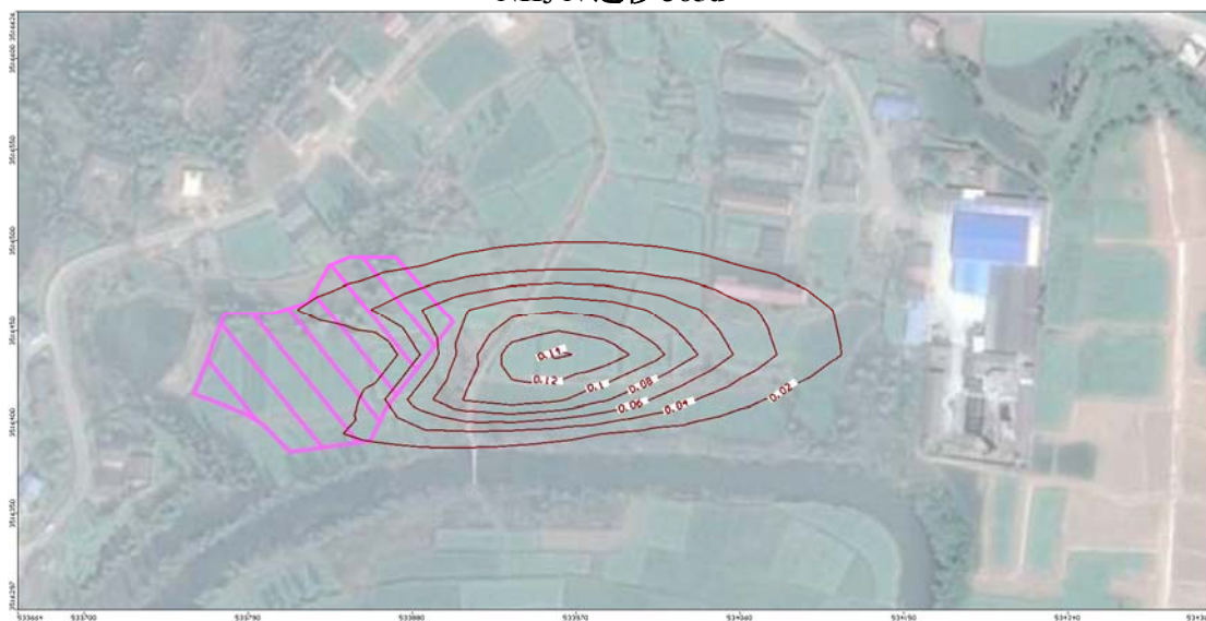
NH 3 -N 迁移 500d
