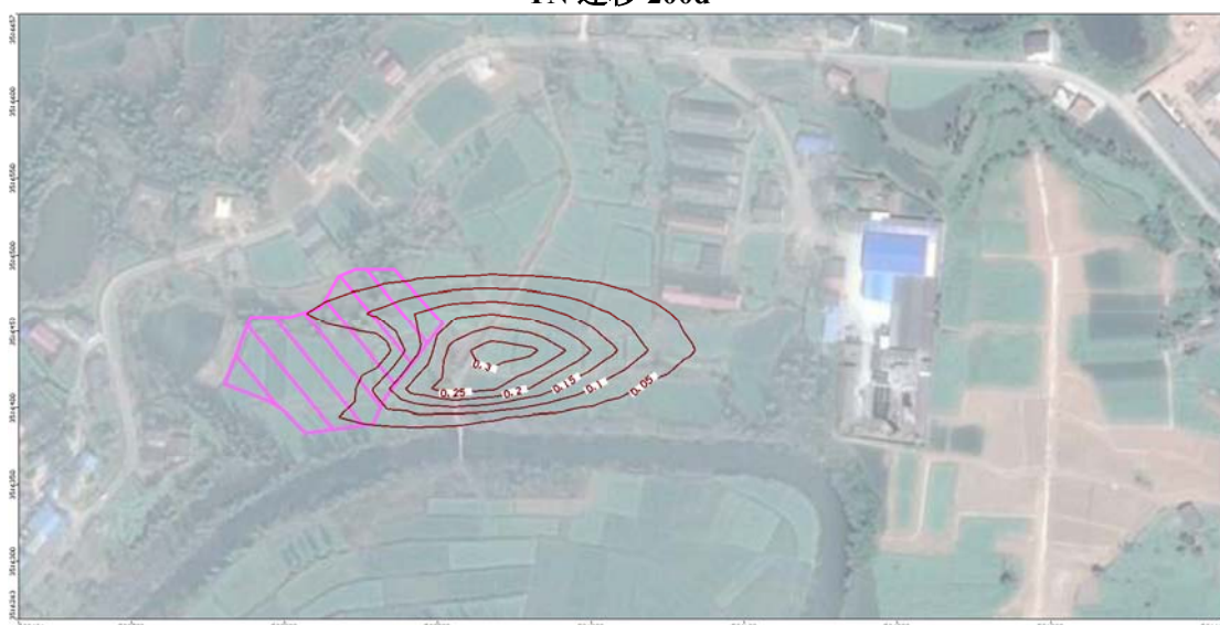
TN 迁移 365d
