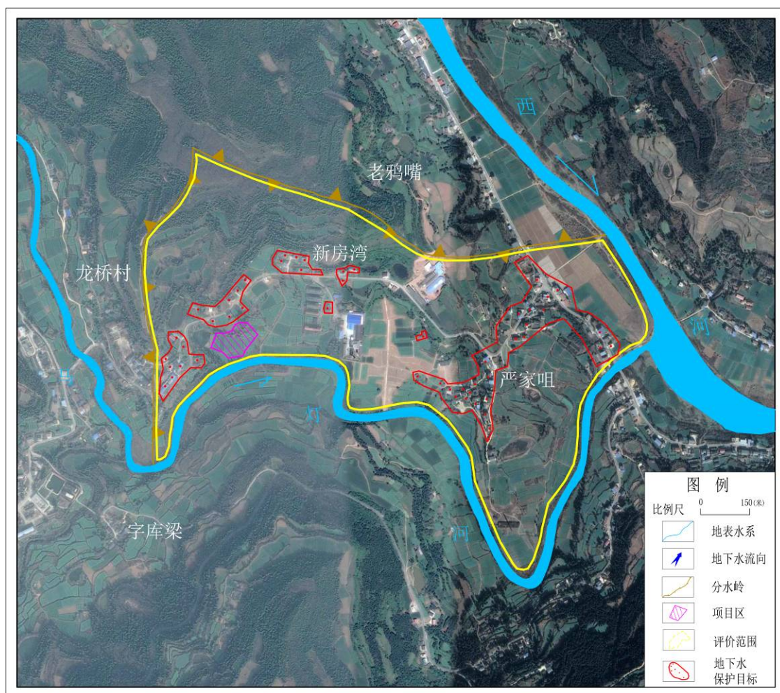
图 1.6-2 地下水环境影响调查评价范围及保护目标图
