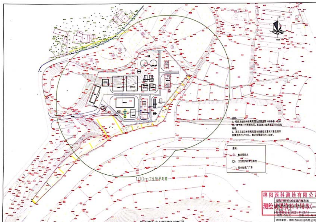
图 5.3-3 项目卫生防护距离包络线图
