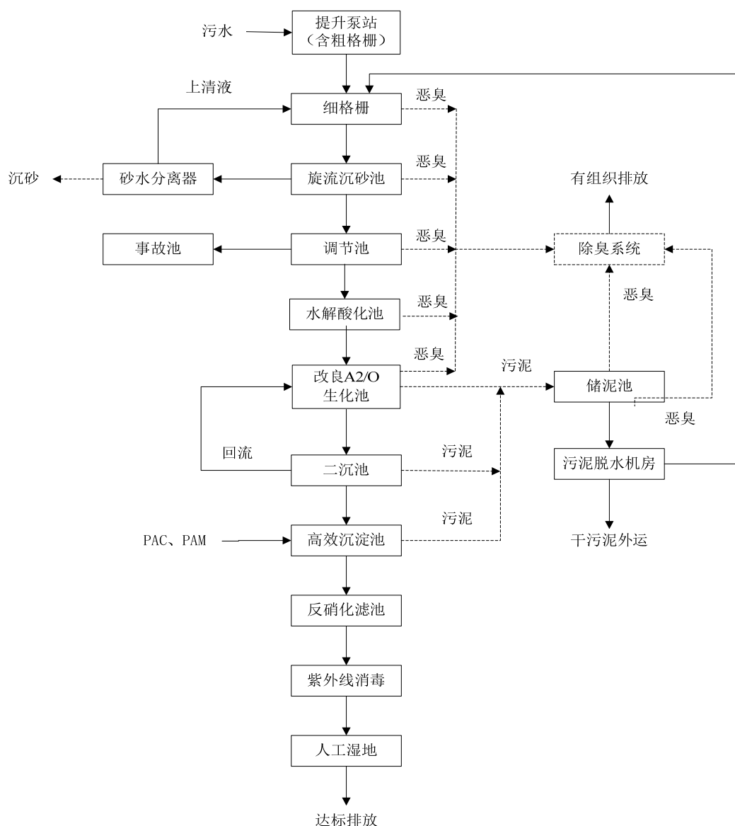
图 2.9-4 项目工艺流程及产污环节图
