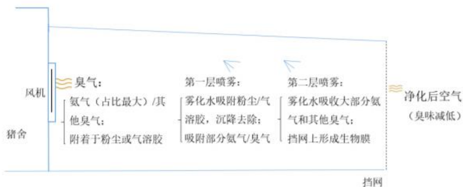
图 6-3 猪舍除臭装置示意图
