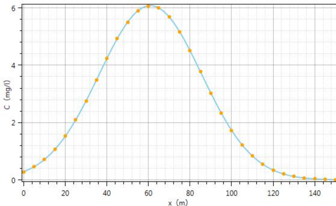
图5.2-6 调节池泄露3650d时氨氮预测结果图
