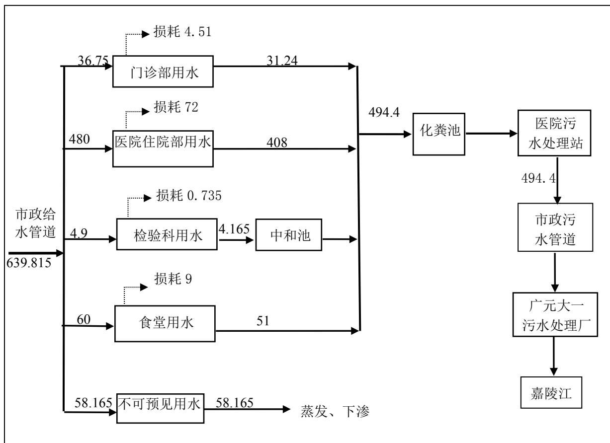
图 3.2-3 项目运营期水平衡图（单位：m 3 /d）
