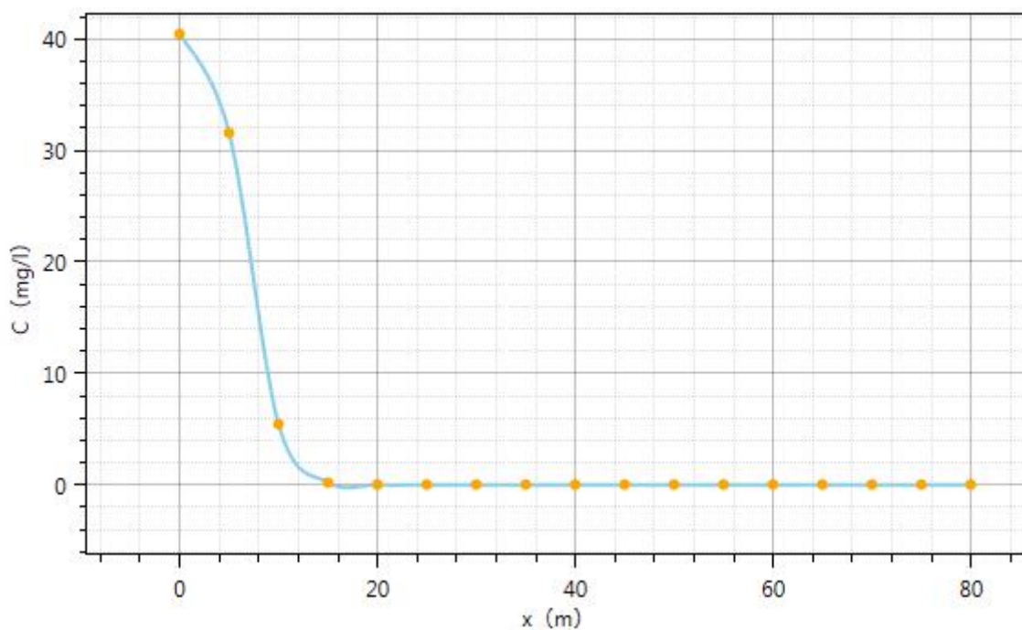
图5.2-1 调节池泄露100d时 COD_{Mn} 预测结果图
