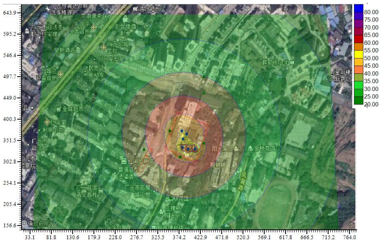
噪声预测等值线图
