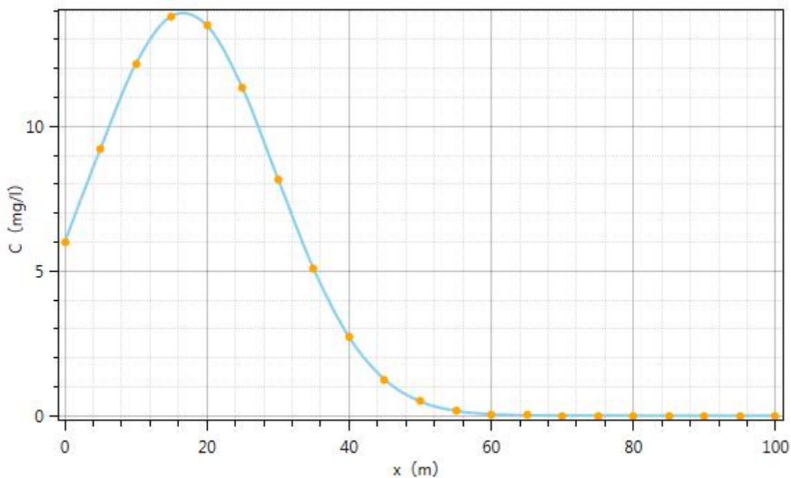
图5.2-2 调节池泄露1000d时COD Mn 预测结果图
