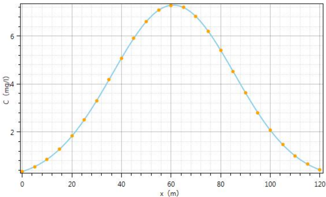
图5.2-3 调节池泄露3650d时COD Mn 预测结果图
