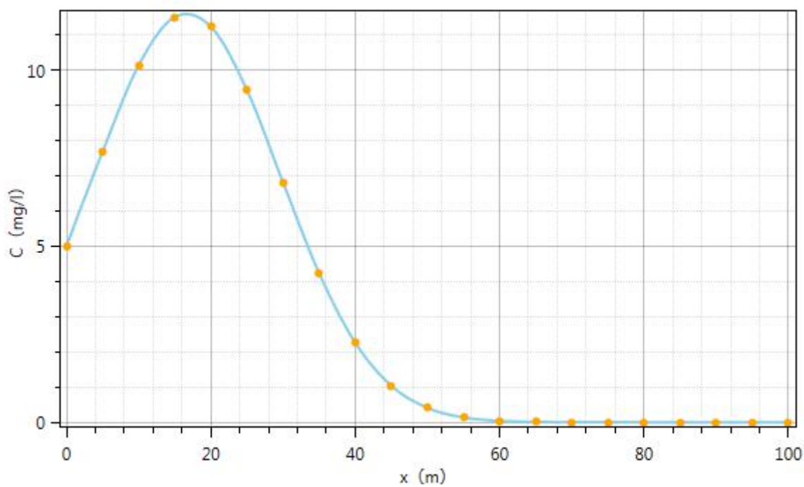
图5.2-5 调节池泄露1000d时氨氮预测结果图
