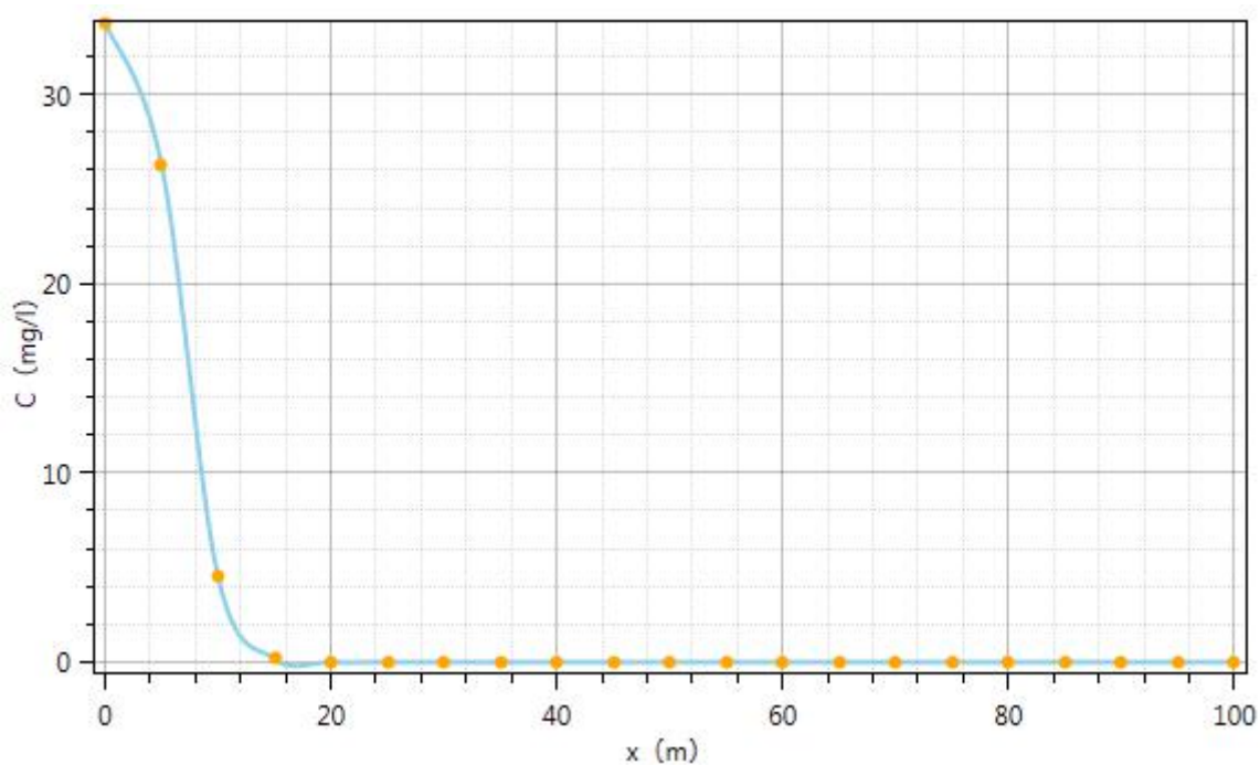
图5.2-4 调节池泄露100d时氨氮预测结果图
