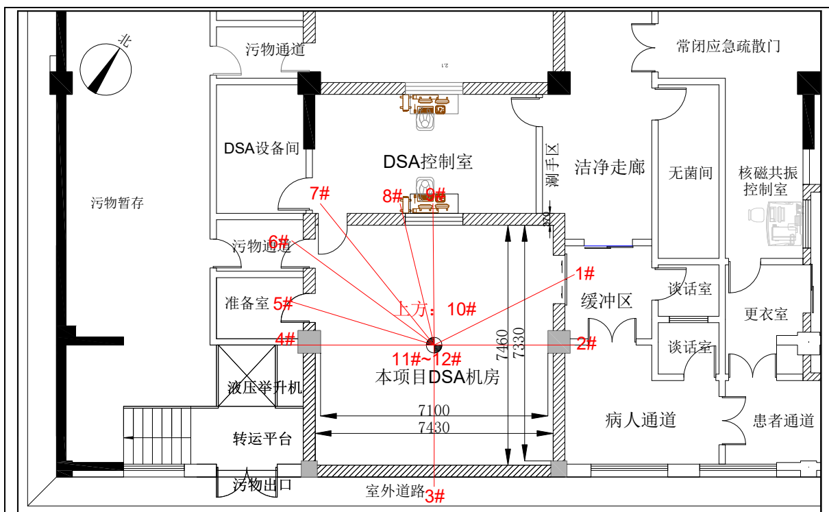
图 11-1 DSA 机房预测点布设示意图
