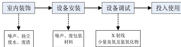
图 9-1 施工期工艺流程及产污环节示意图
