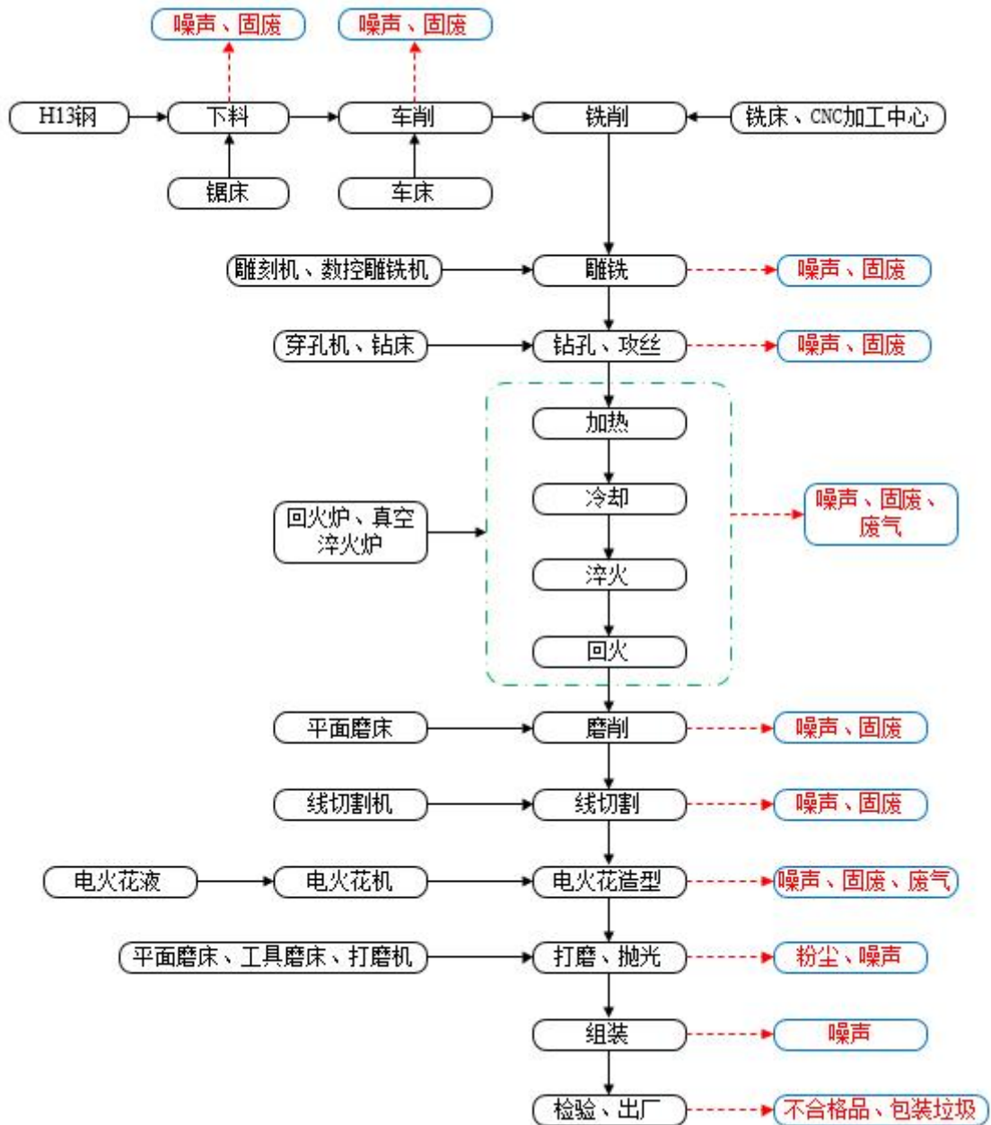
图 2-2 运营期工艺流程及产污位置示意图
