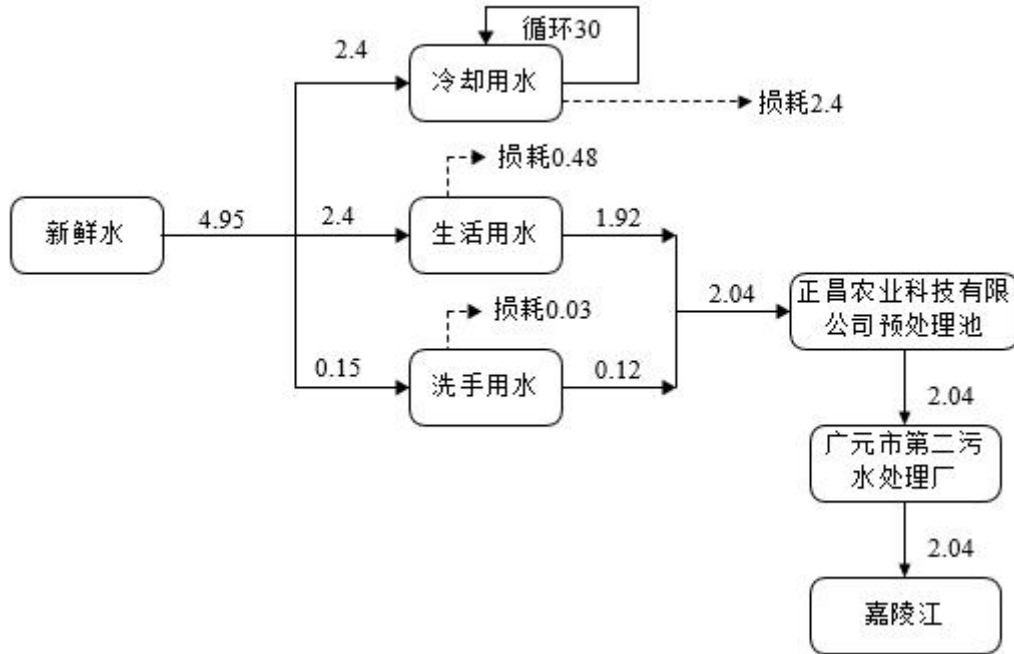
图 2-4 项目营运期水量平衡示意图 单位：m 3 /d
