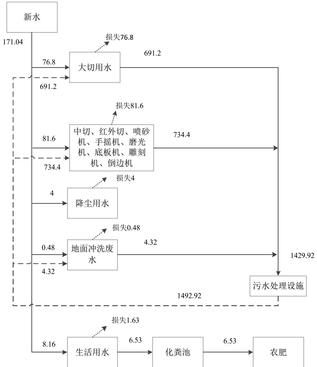
图2-1 全厂水平衡图 单位：m 3 /d
