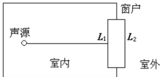
图 4-2 室内声源等效为室外声源图
