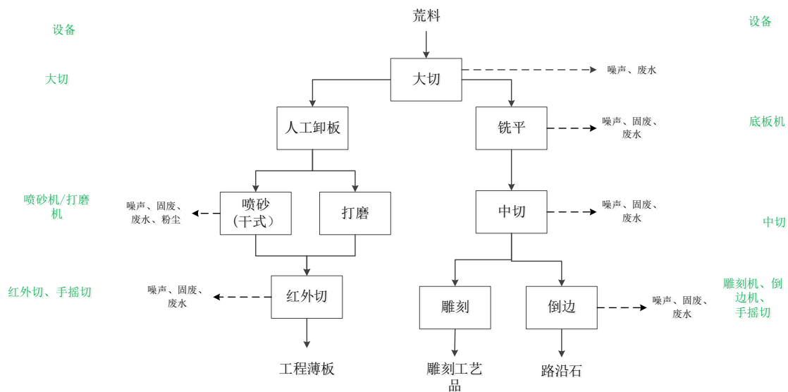
图 2-3 项目工艺流程及产污环节图
