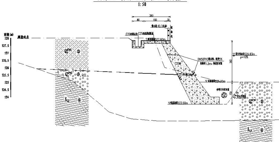
方案二：仰斜式挡墙（比较堤型）
