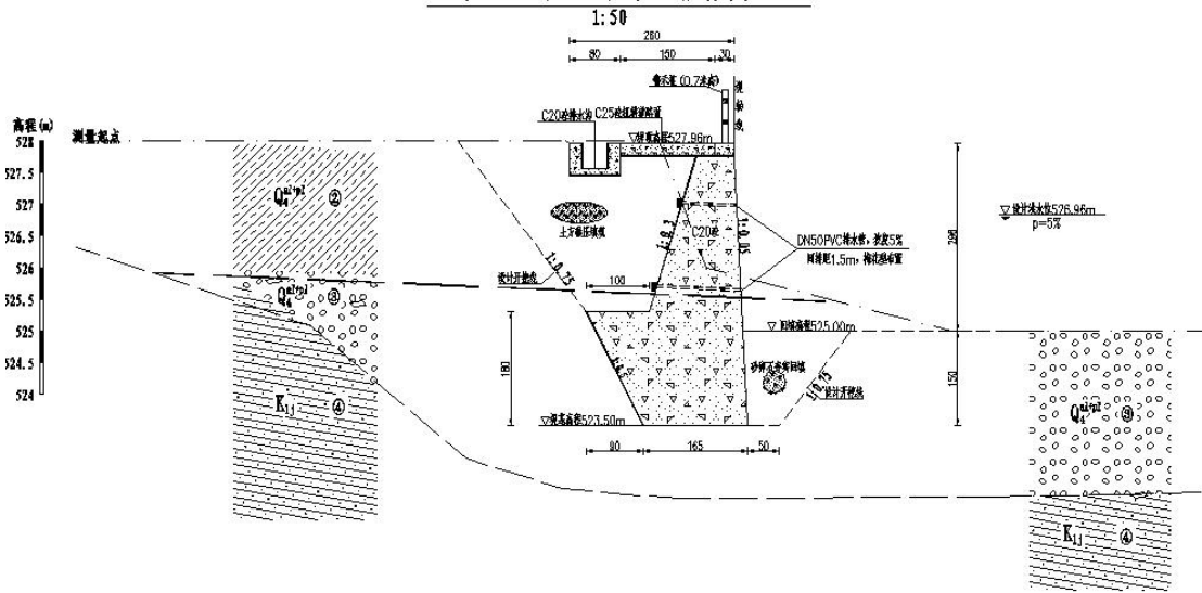
方案一：衡重式挡墙（推荐堤型）
