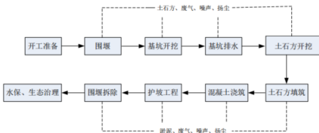
图 2-5 防洪堤修建工艺流程图
