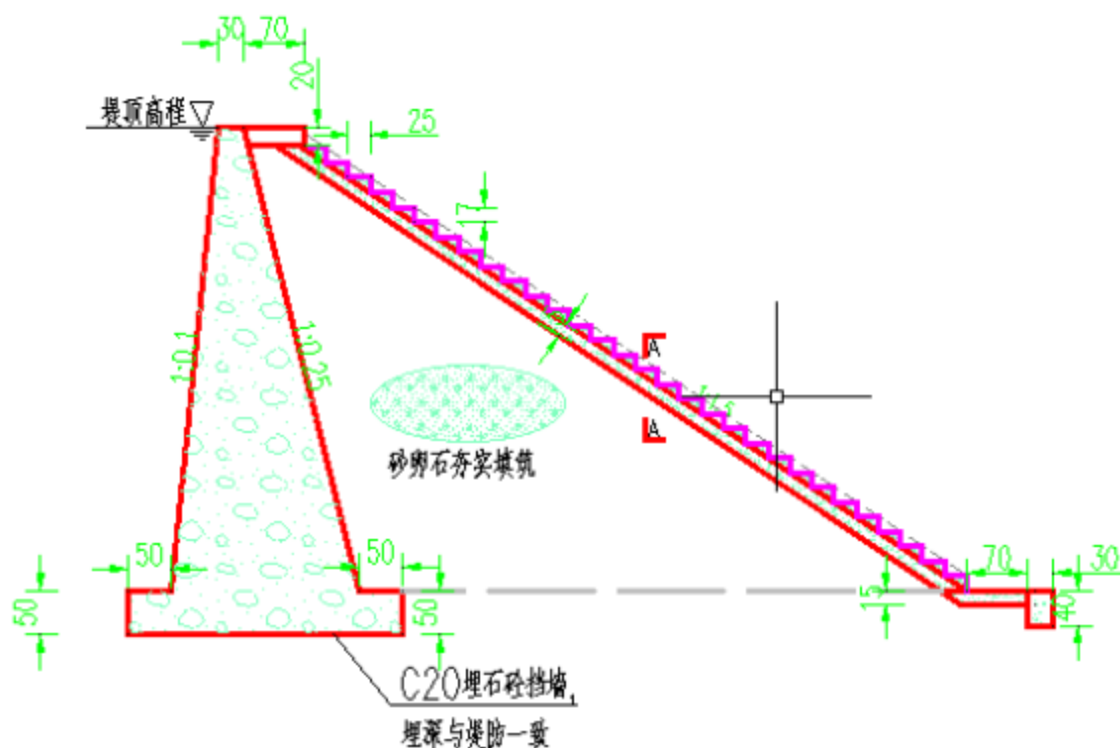
图 2-4 下河梯步典型横断面
