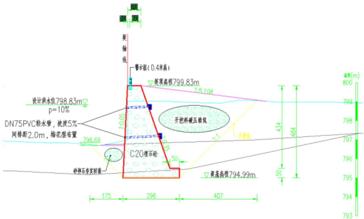
图 2-1 新建重力式堤防结构典型横断面
