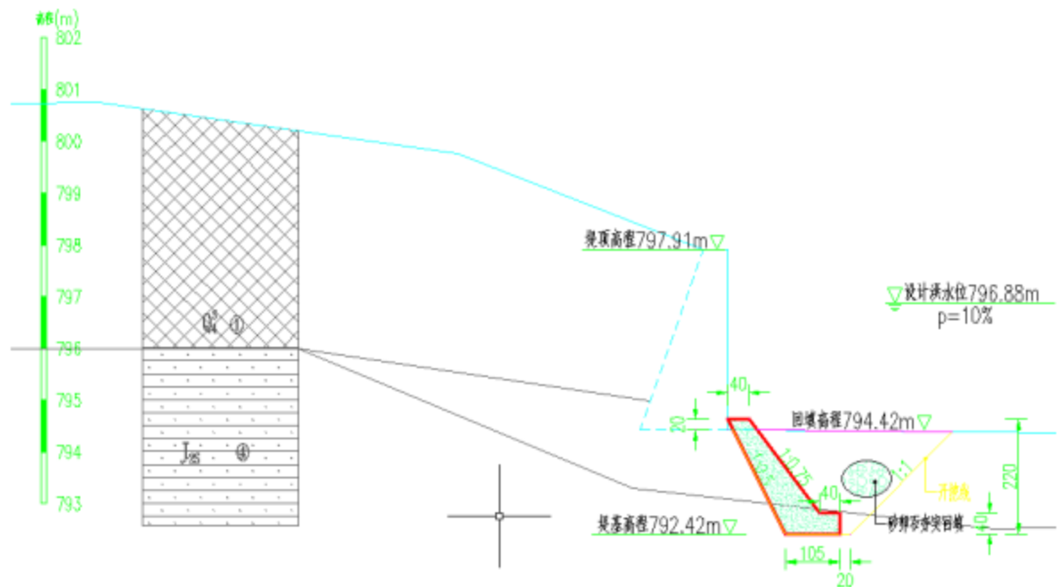
图 2-2 加固段仰斜式护脚结构典型横断面
