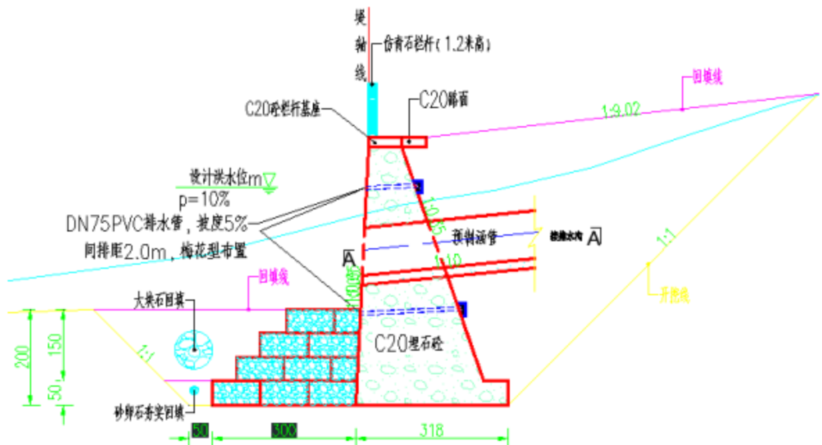
图 2-3 穿堤涵管结构典型横断面
