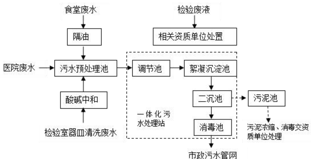
图 2.6-1 现污水处理站工艺流程图
