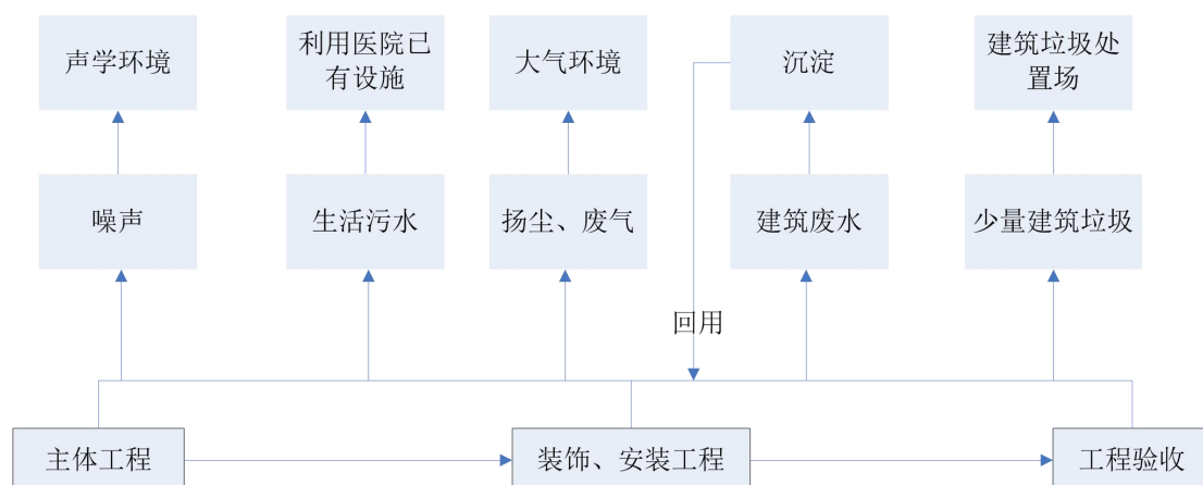
图 4.1-1 施工期工艺流程及产污环节图
