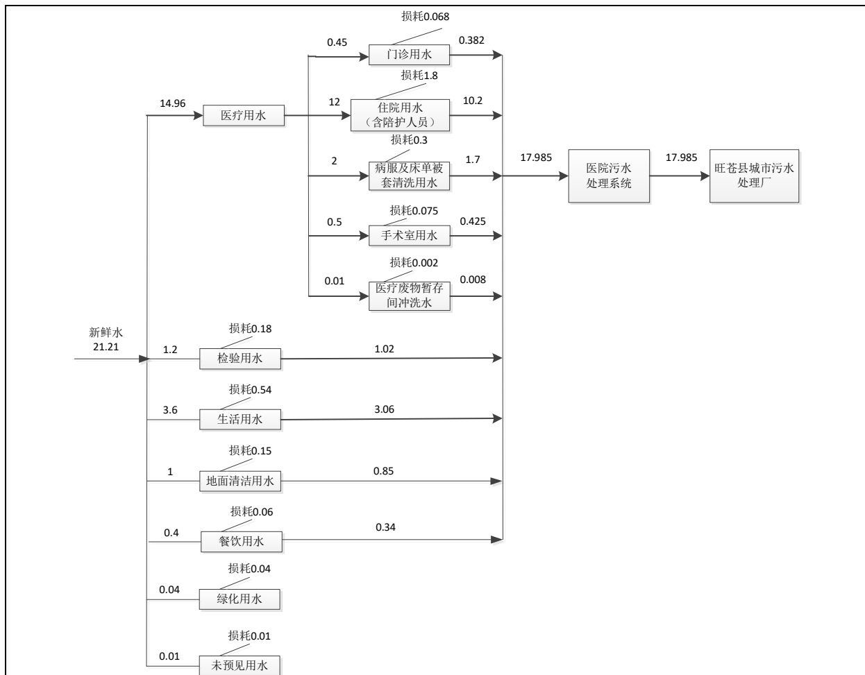
图 5-2 项目水平衡图 单位: m³/d
