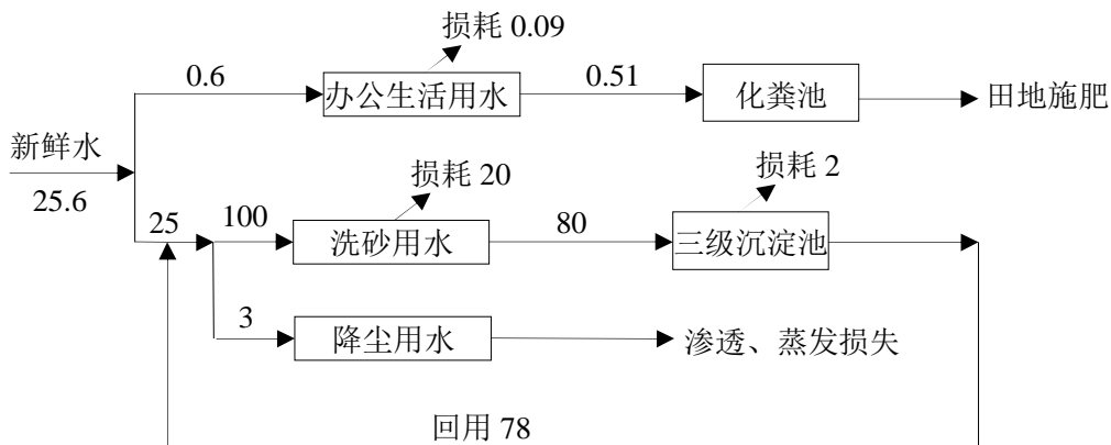
图 5-2 项目水平衡图 单位 m 3 /d
