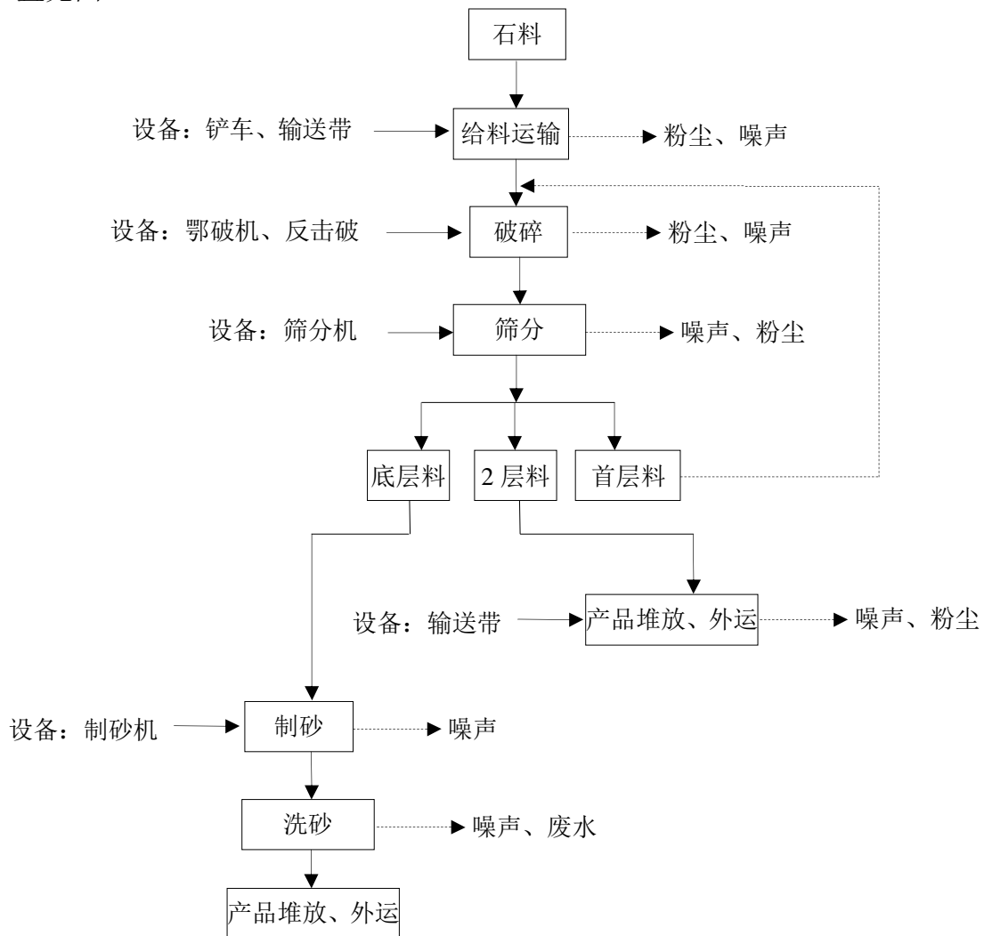
图 5-1 营运期生产工艺流程及产污位置图
