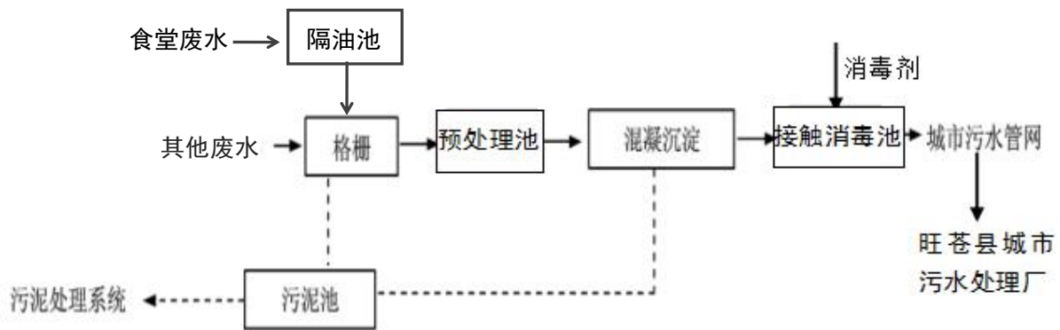
图 5-3 废水处理工艺流程
