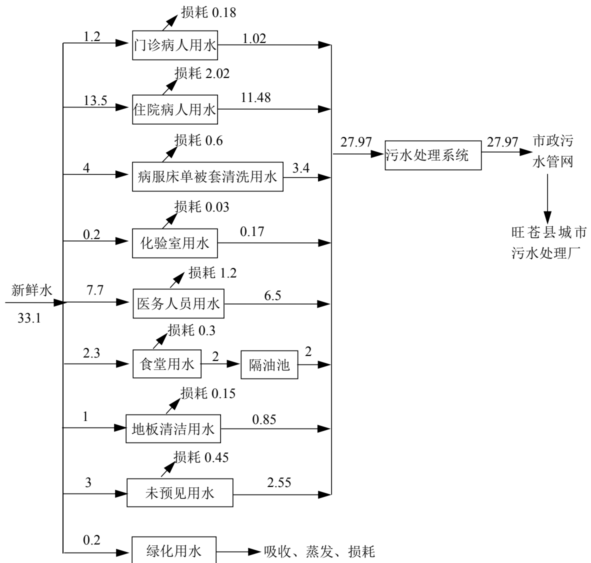
图 5-2 项目水平衡图 (单位 \text{m}^3/\text{d} )
