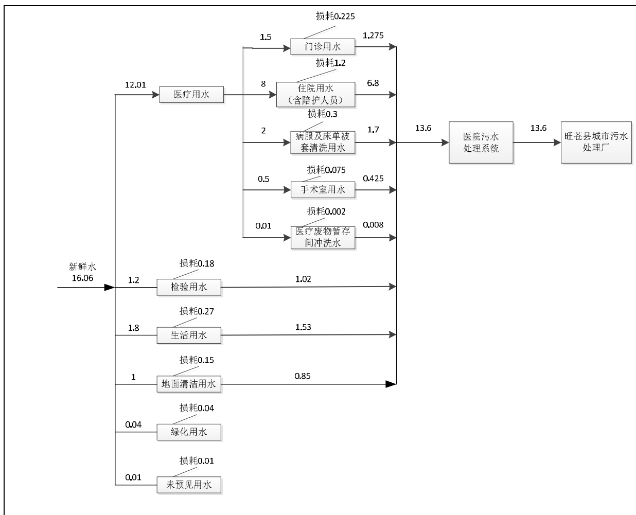
图 5-2 项目水平衡图 单位: \text{m}^3/\text{d}
