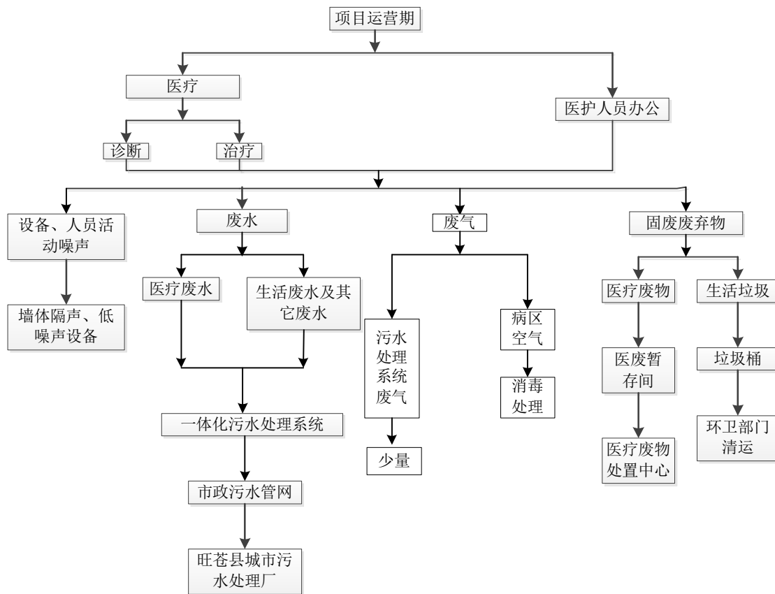
图 5-1 项目运营期流程及产污位置示意图
