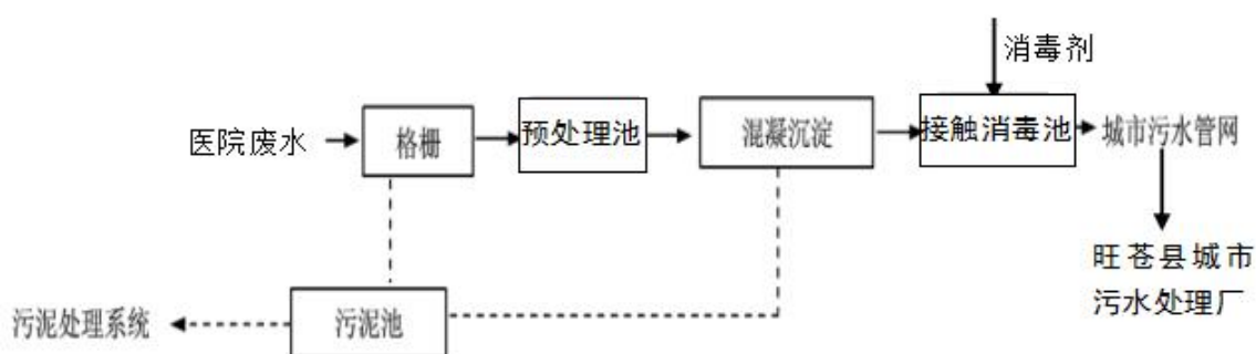
图 5-3 改造后废水处理工艺流程
