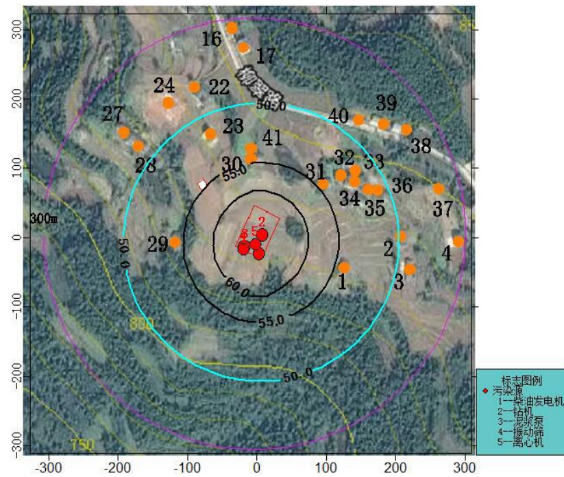
图 7-2 钻井作业夜间噪声预测等声级图（声级单位：dB(A)）
