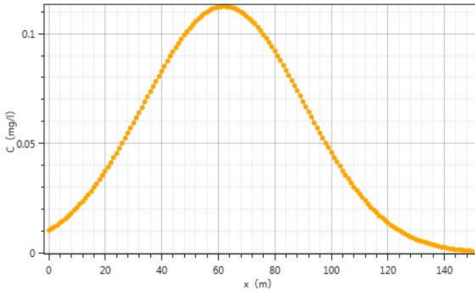
图 4-2 污染后 365 天水流下游轴向污染物浓度变化趋势图
