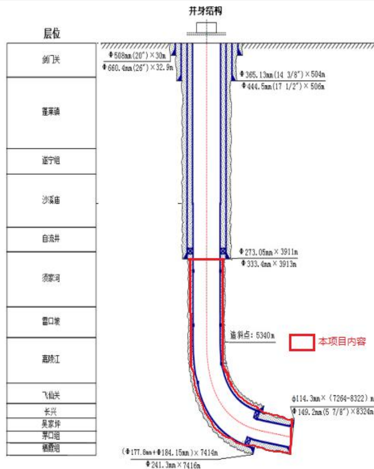
图 5-3 井身结构示意图
