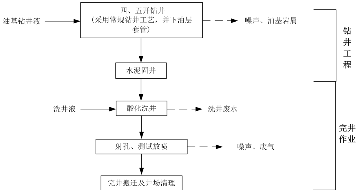
图 5-2 项目工程作业流程及产污环节图
