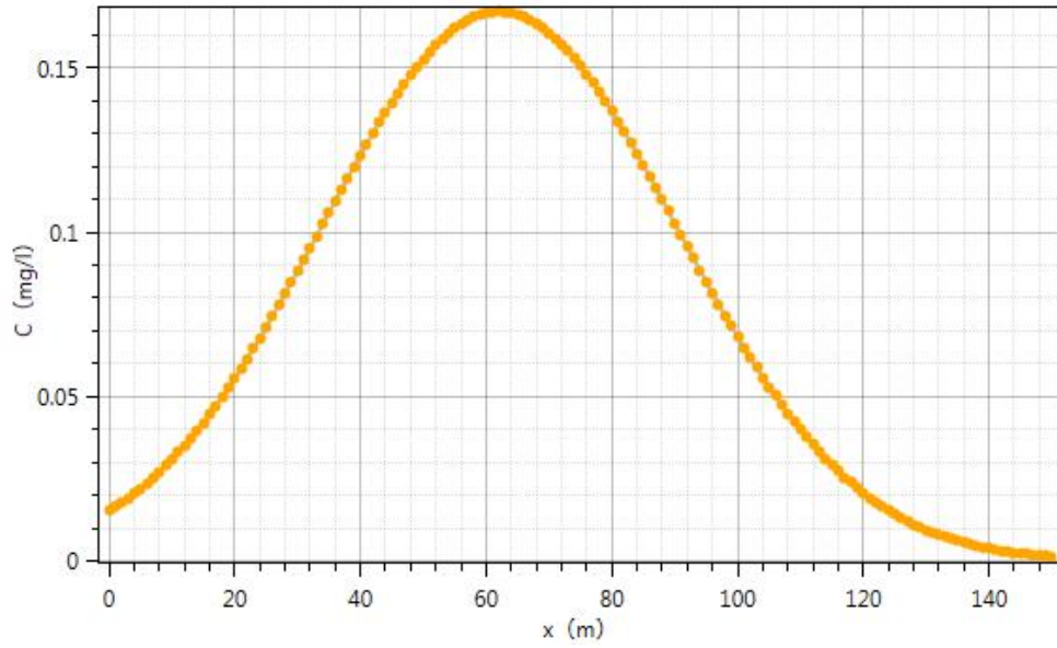
图 4-8 污染后 365 天水流下游轴向污染物浓度变化趋势图
