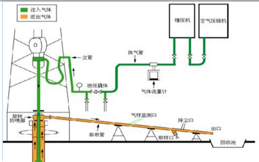
图 1-17 空气钻井阶段作业流程图
