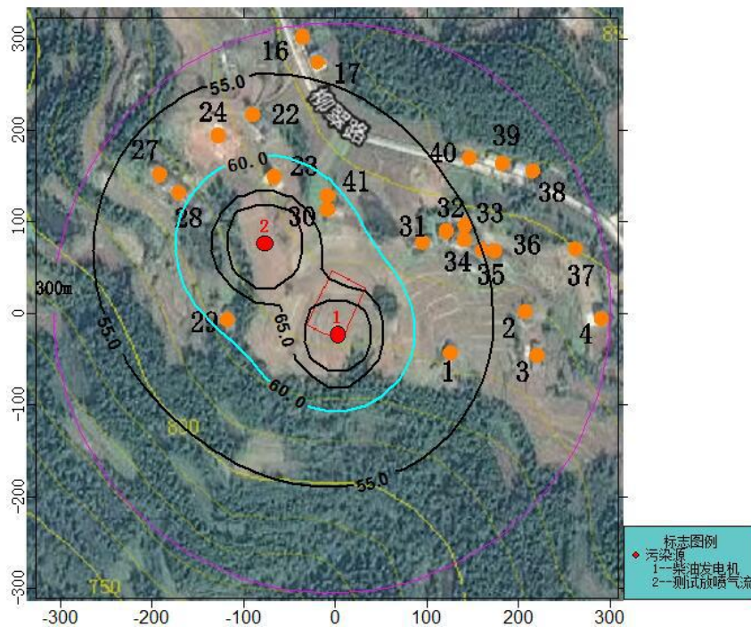
图 7-3 测试放喷期间昼间噪声预测等声级图（声级单位：dB(A)）
