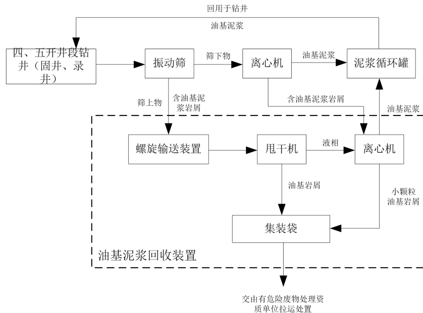
图 5-4 油基钻井液钻阶段作业流程及产污节点图
