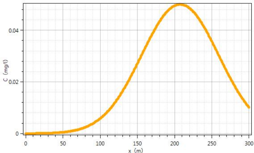
图 4-11 污染后 1220 天水流下游轴向污染物浓度变化趋势图
