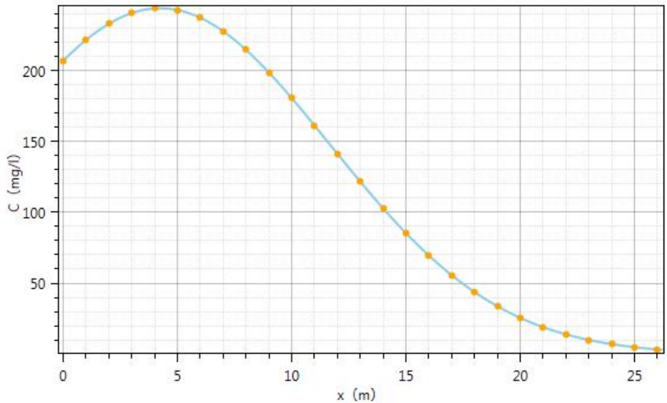
图 4-13 污染后 25 天水流下游轴向污染物浓度变化趋势图
