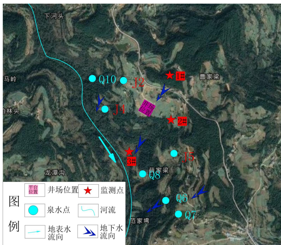
图 5-1 地下水环境跟踪监测布点示意图
