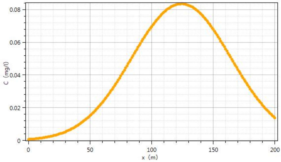
图 4-9 污染后 730 天水流下游轴向污染物浓度变化趋势图
