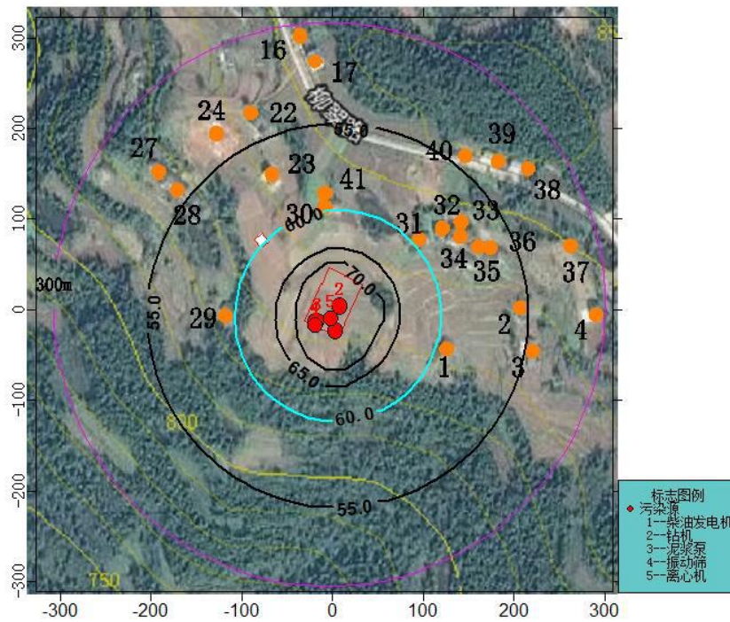
图 7-1 钻井作业昼间噪声预测等声级图（声级单位：dB(A)）
