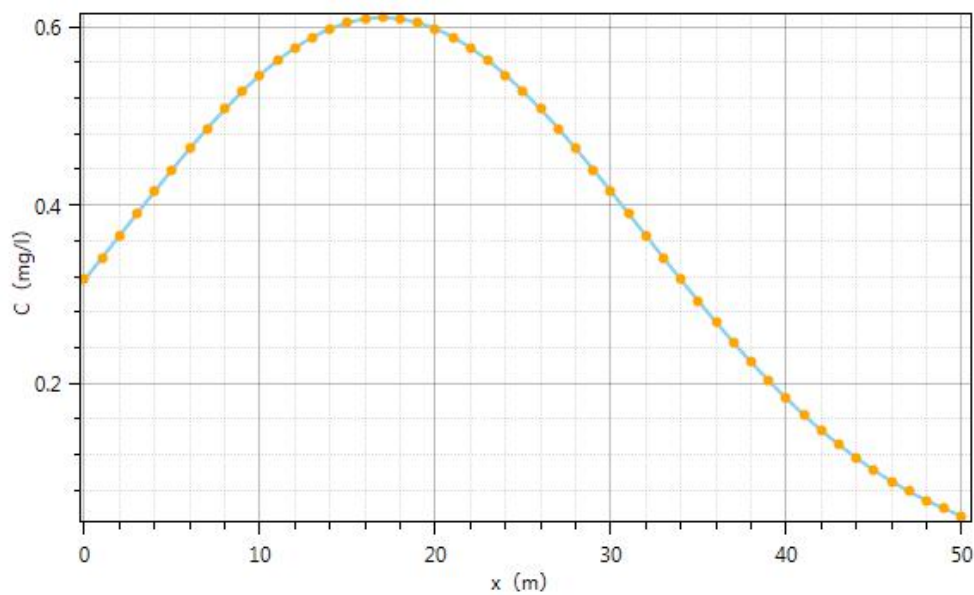
图 4-7 污染后 100 天水流下游轴向污染物浓度变化趋势图
