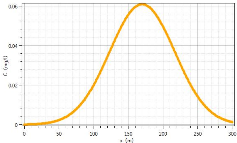
图 4-10 污染后 1000 天水流下游轴向污染物浓度变化趋势图
