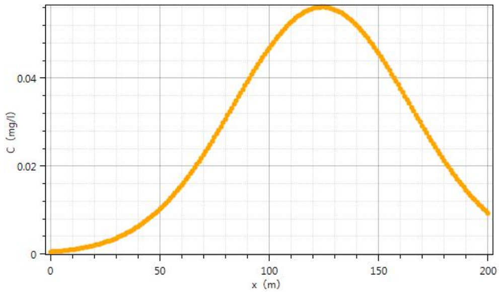
图 4-3 污染后 730 天水流下游轴向污染物浓度变化趋势图
