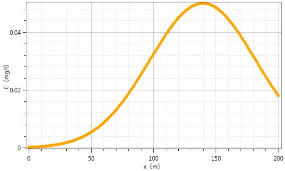
图 4-4 污染后 820 天水流下游轴向污染物浓度变化趋势图
