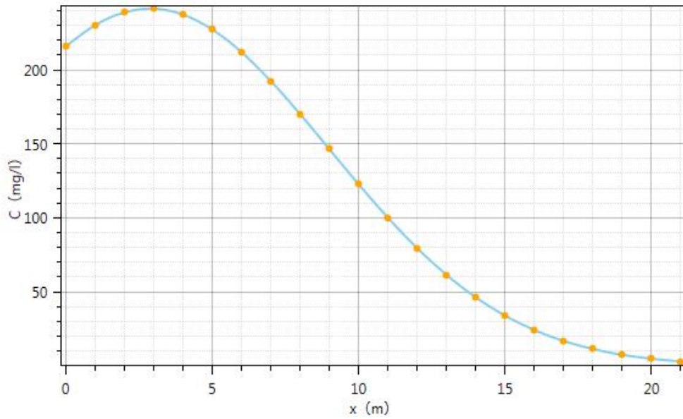
图 4-6 污染后 17 天水流下游轴向污染物浓度变化趋势图
