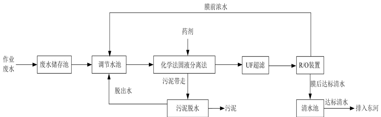
图 5-6 四川鑫泓废水处理有限公司废水处理工艺流程示意图
